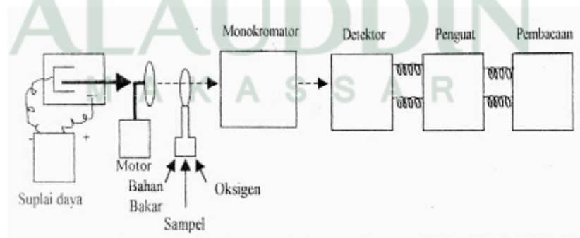
Gambar . skema alat Spektrofotometer Serapan Atom
