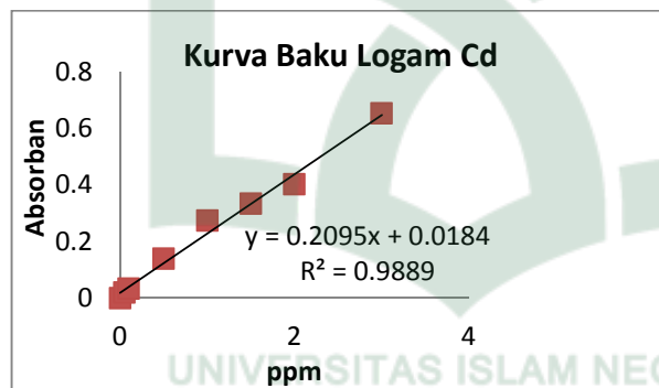
Gambar 11. Kurva baku logam Kadmium (Cd)
