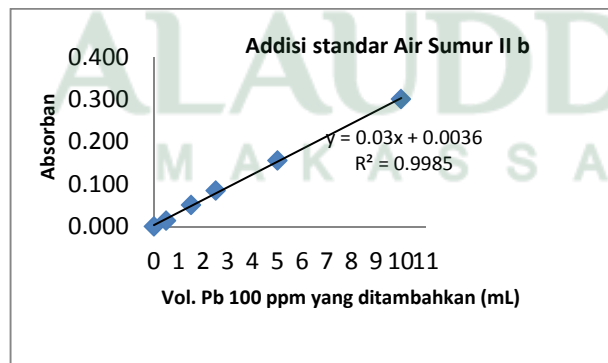
Gambar 6. Kurva addisi standar sumur 2 (b)
