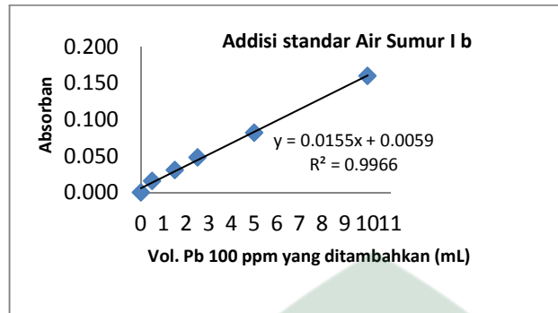
Gambar 3. Kurva addisi standar sumur 1 (b)
