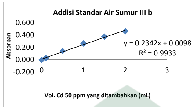
Gambar 19. Kurva addisi standar sumur 3 (b)
