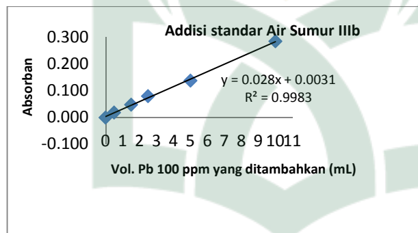
Gambar 9. Kurva addisi standar sumur 3 (b)
