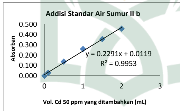
Gambar 16. Kurva addisi standar sumur 2 (b)
