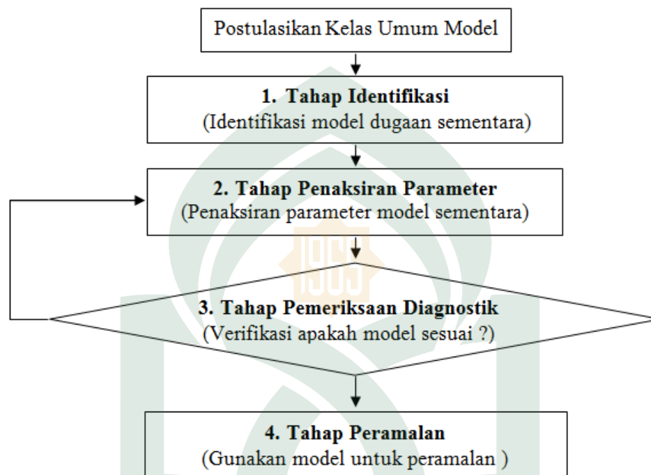
Gambar 2.1 Skema yang memperlihatkan pendekatan Box-Jenkins 17
