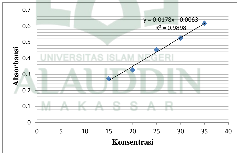
Gambar 5. Kurva Baku Nifedipin
