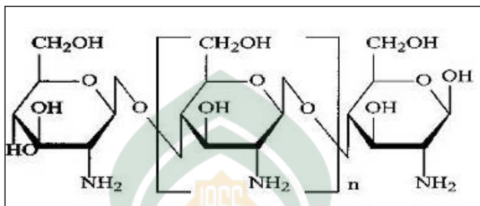
Gambar 4. Struktur Kimia Senyawa Kitosan (Nair et al , 2009 : 1).
