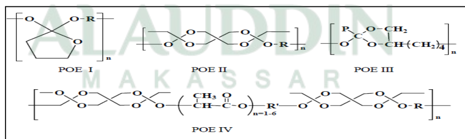
Gambar 3. Struktur kimia senyawa poli ortho ester ( Park et al , 2005 : 7)
