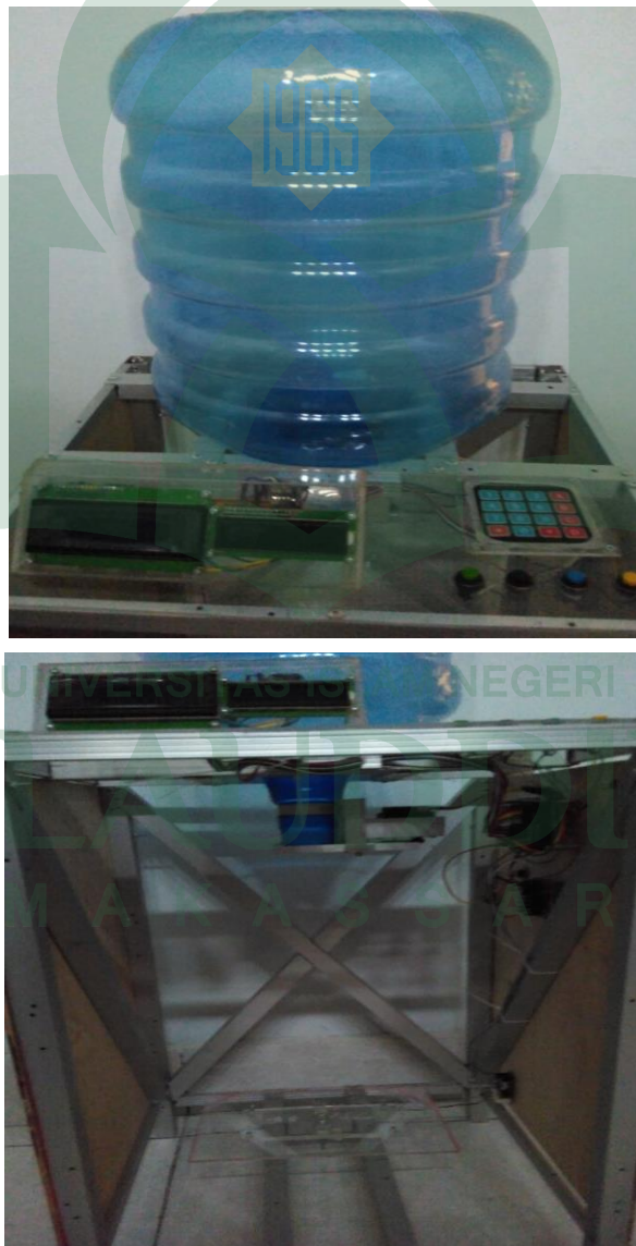
Gambar V.1 Hasil Rancangan Alat Secara Keseluruhan.
