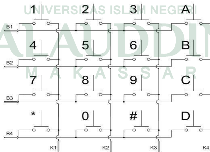
Gambar IV.6 Rangkaian Keypad (Chandra, 2015).
