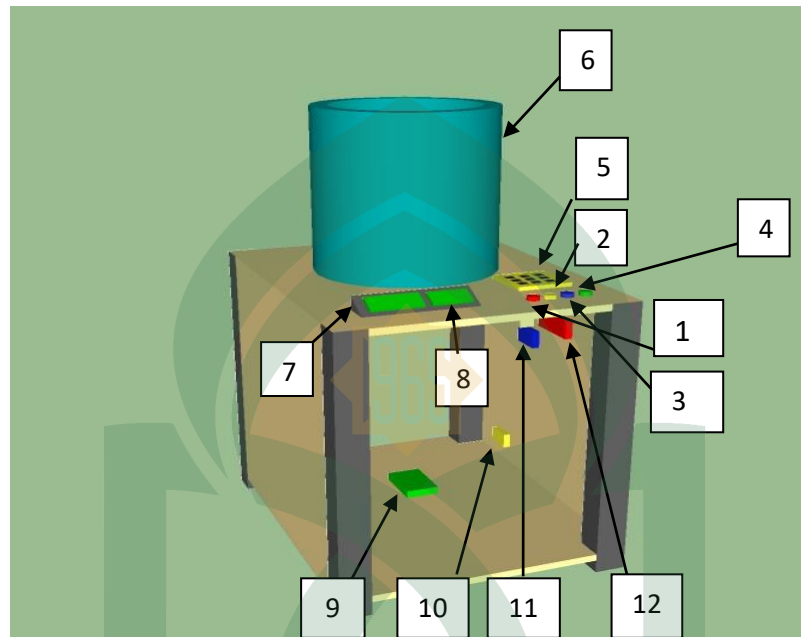
Gambar IV.2 Rancangan Bentuk Fisik Timbangan.
