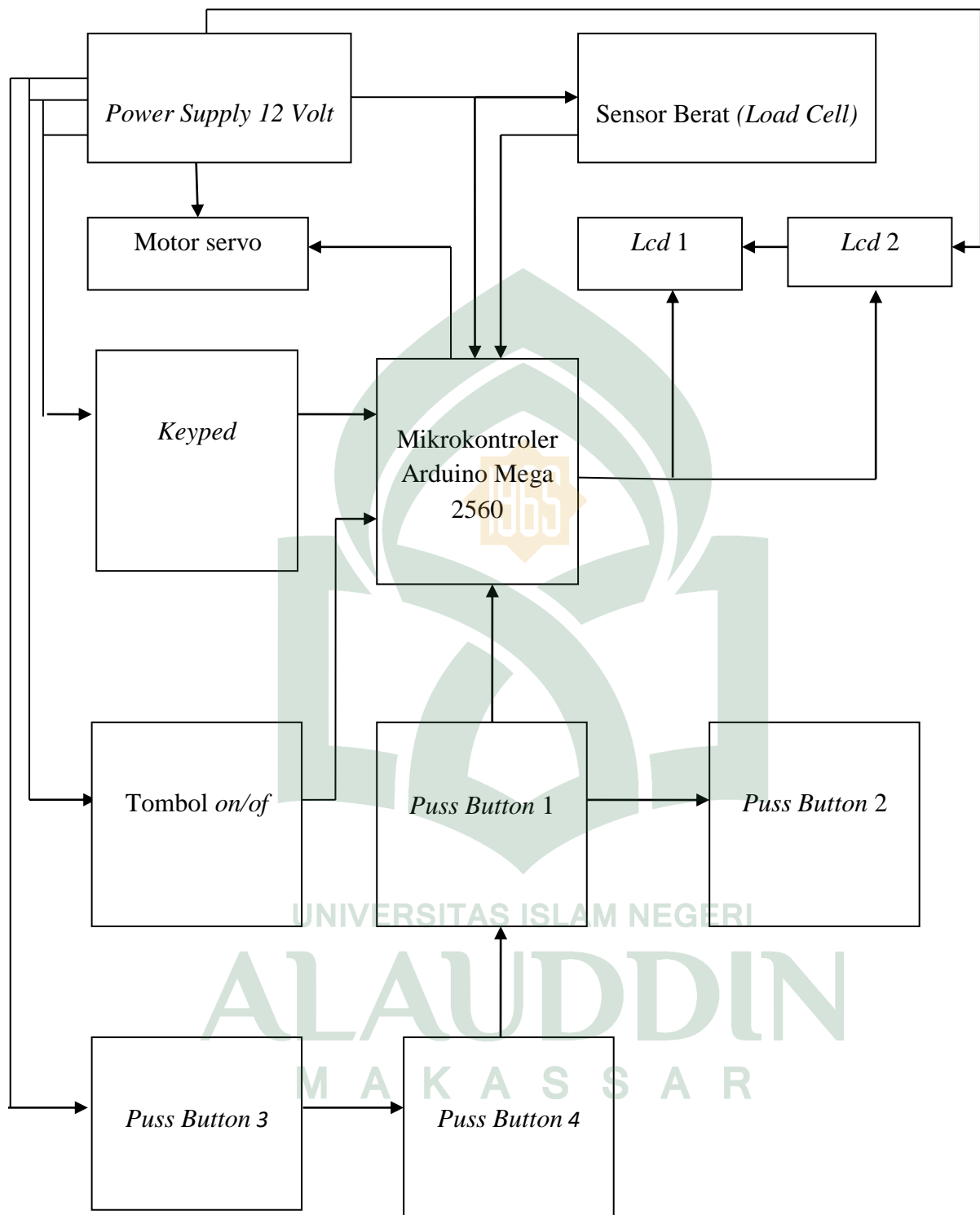
Gambar IV.1 Diagram Blok Rancang Bangun Timbangan Beras Digital dengan Keluaran Berat dan Harga Berbasis Mikrokontroler.
