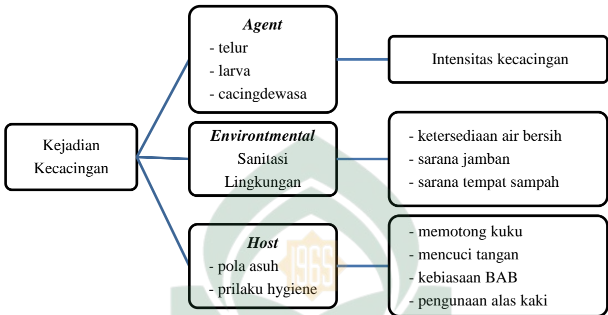
Gambar 2.1 : Kerangka Teori
