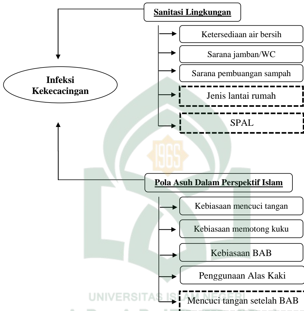
Gambar 2.2 : Kerangka Pikir
