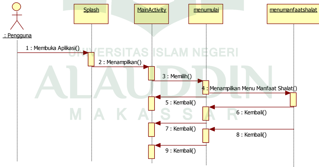
Gambar IV.12. Sequence Diagram Menampilkan Menu Manfaat Gerakan Shalat
