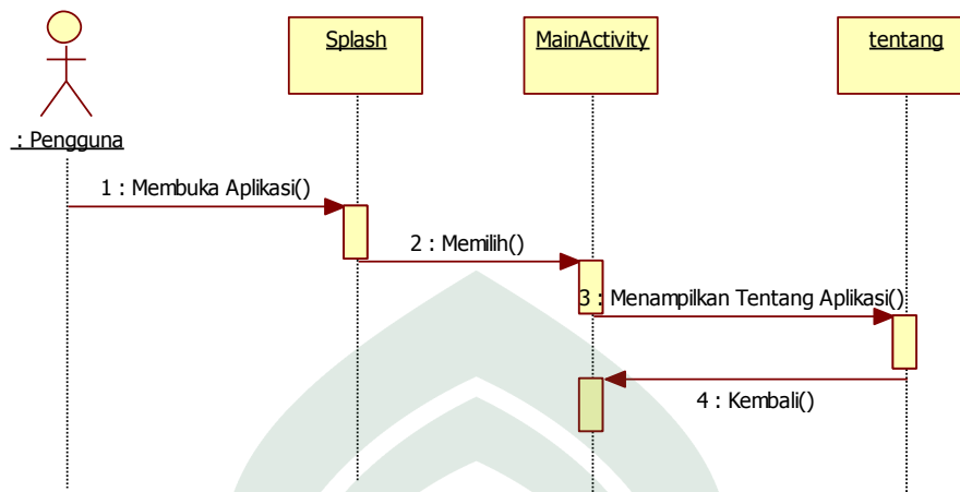
Gambar IV.5. Sequence Diagram Menampilkan Menu Tentang Aplikasi
