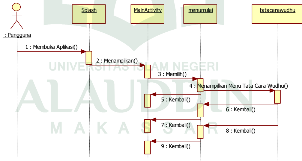
Gambar IV.14. Sequence Diagram Menampilkan Menu Tata Cara Wudhu
