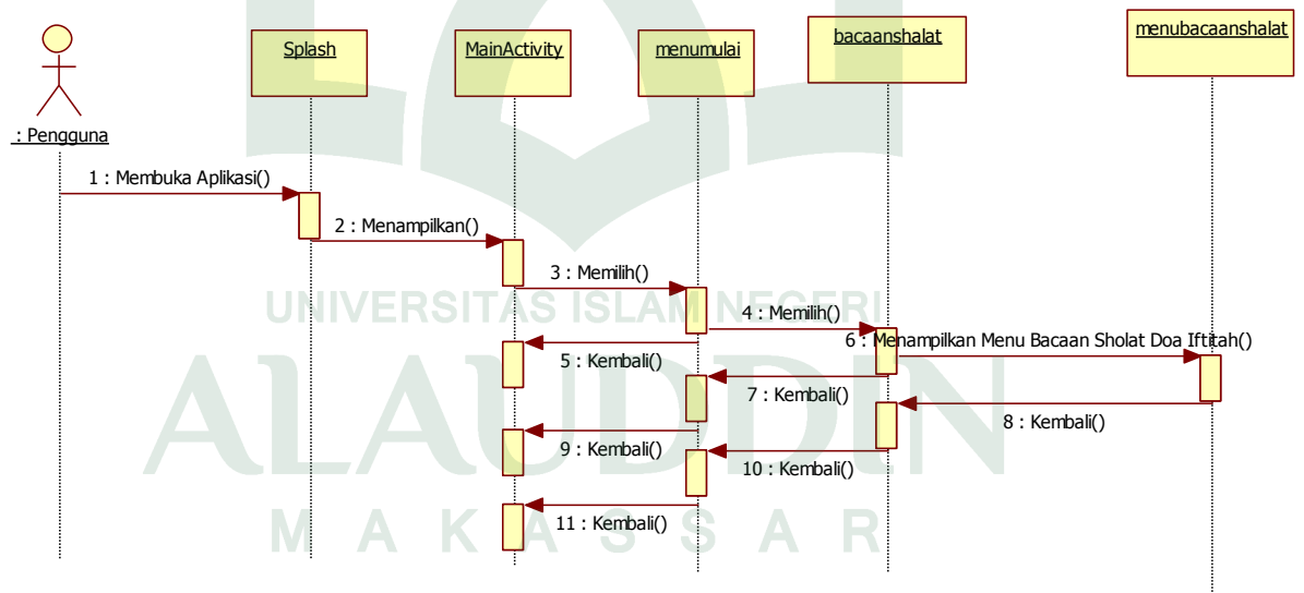
Gambar IV.10. Sequence Diagram Menampilkan Menu Bacaan Shalat Do'a
