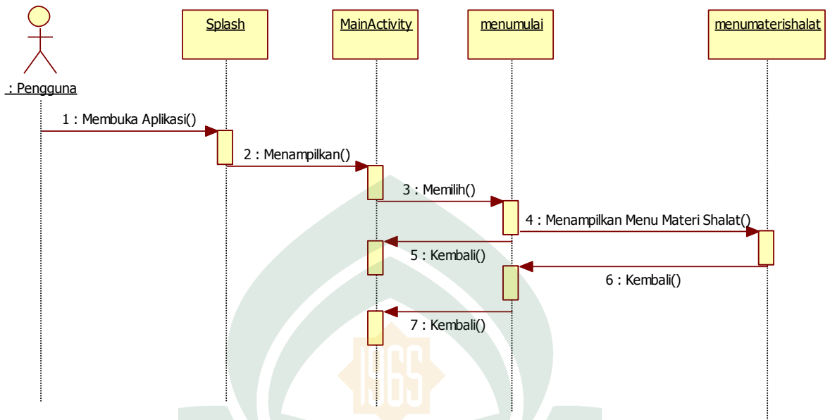
Gambar IV.7. Sequence Diagram Menampilkan Menu Materi Shalat
