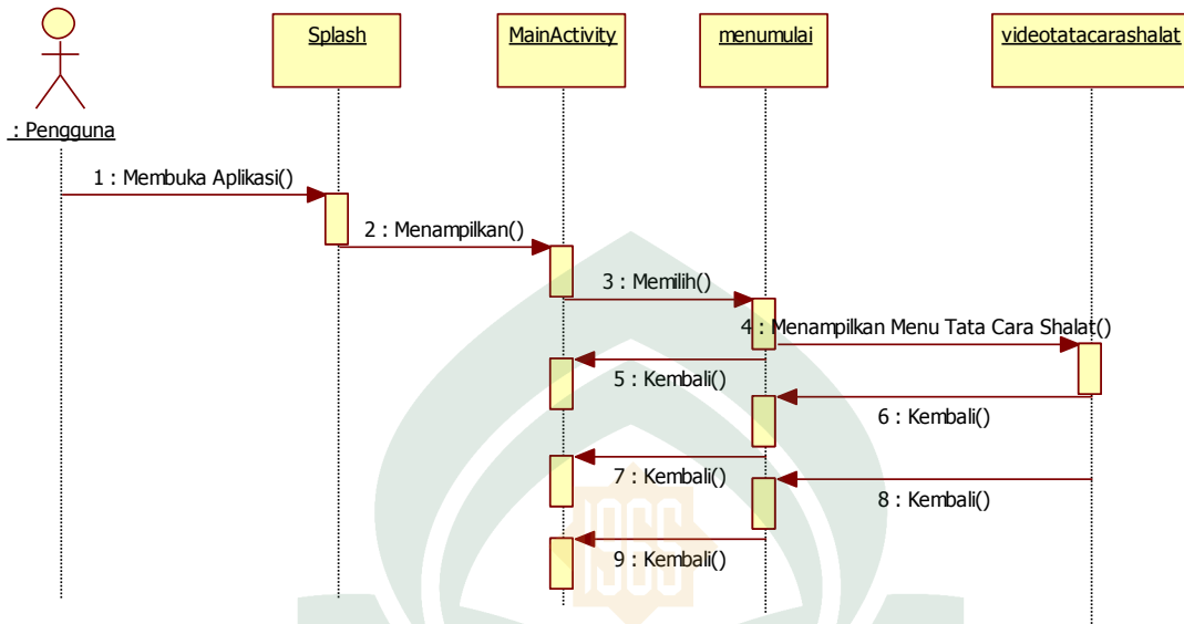
Gambar IV.11. Sequence Diagram Menampilkan Menu Tata Cara Shalat
