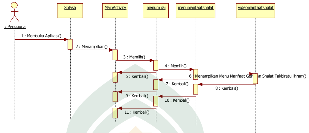
Gambar IV.13. Sequence Diagram Menampilkan Menu Manfaat Gerakan Shalat Takbiratul Ihram
