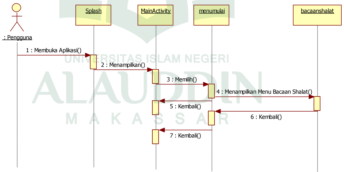
Gambar IV.8. Sequence Diagram Menampilkan Menu Bacaan Shalat
