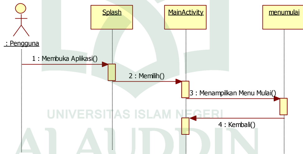
Gambar IV.6. Sequence Diagram Menampilkan Menu Mulai
