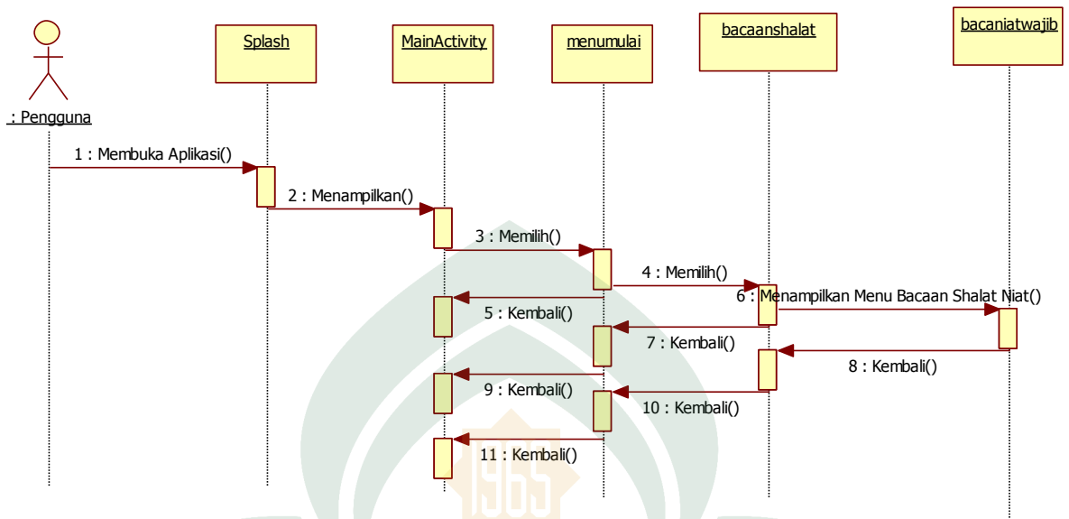
Gambar IV.9. Sequence Diagram Menampilkan Menu Bacaan Niat Shalat
