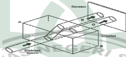
Gambar 2.13 Polarisasi Karena Pembiasan Rangkap
