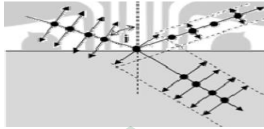
Gambar 2.11 Proyeksi Getaran Elektron Untuk Sudut Datang Sembarang
