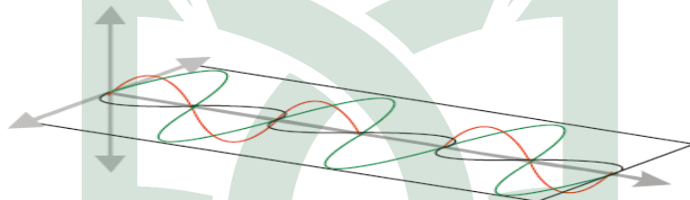
Gambar 2.1 Gelombang Tak Terpolarisasi Pada Tali
