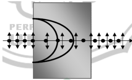
Gambar 2.16 Permukaan Kristal Dipotong Seajar Sumbu Optis.
