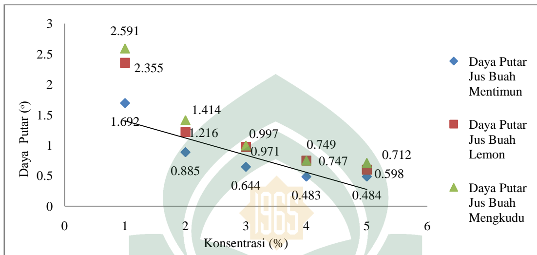
Grafik 4.1.2 Hubungan Antara Konsentrasi dan Daya Putar Terhadap Sifat Optik Aktif dari Jus Buah Mentimun, Lemon dan Mengkudu.
