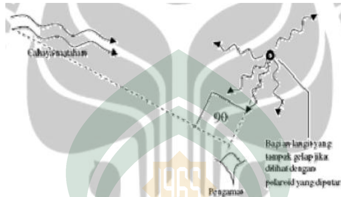
Gambar 2.18 Cahaya Matahari Dihamburkan Oleh Partikel-Partikel Udara
