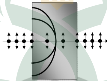
Gambar 2.15 Permukaan Kristal Dipotong Tegak Lurus Sumbu Optis
