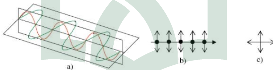
Gambar 2.5 Bentuk Penyederhanaan Gelombang Cahaya Tak Terpolarisasi
