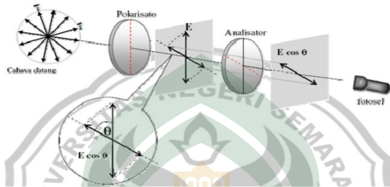
Gambar 2.8 Desain Percobaan Untuk Menganalisis Cahaya Terpolarisasi
