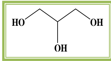
Gambar 2.6 Struktur Gliserin
