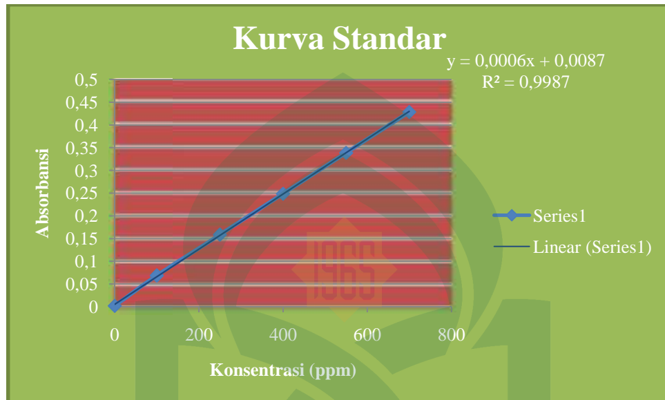
Gambar 4.1 Grafik hubungan antara konsentrasi dengan daya adsorpsi larutan standar kalsium ( \text{Ca}^{2+} )
