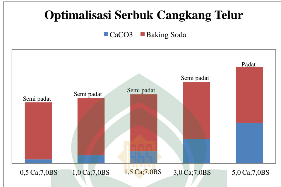
Gambar 4.3 Optimalisasi serbuk cangkang (kalsium karbonat) dalam pembuatan pasta komposit
