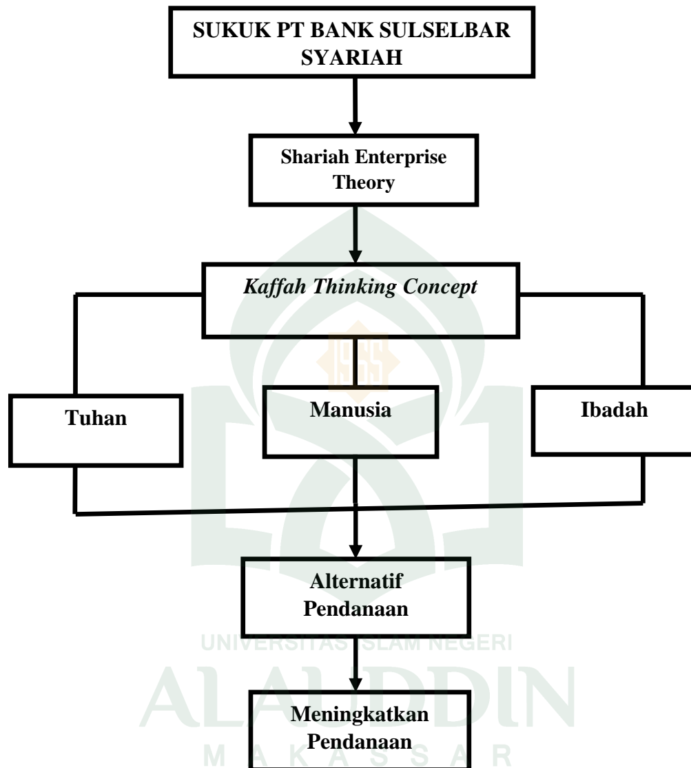
Gambar 2.3 Kerangka Pikir
