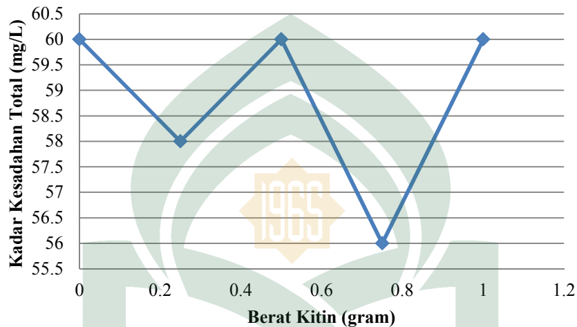
Gambar 4.3 Grafik Hasil Uji Kesadahan pada Air Sungai setelah Penambahan Kitin
