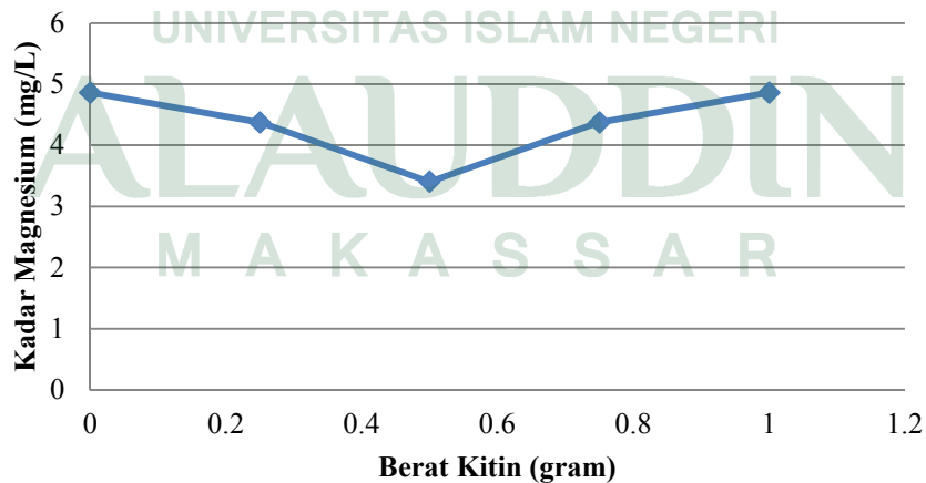
Gambar 4.5 Grafik Hasil Uji Magnesium pada Air Sungai setelah Penambahan Kitin
