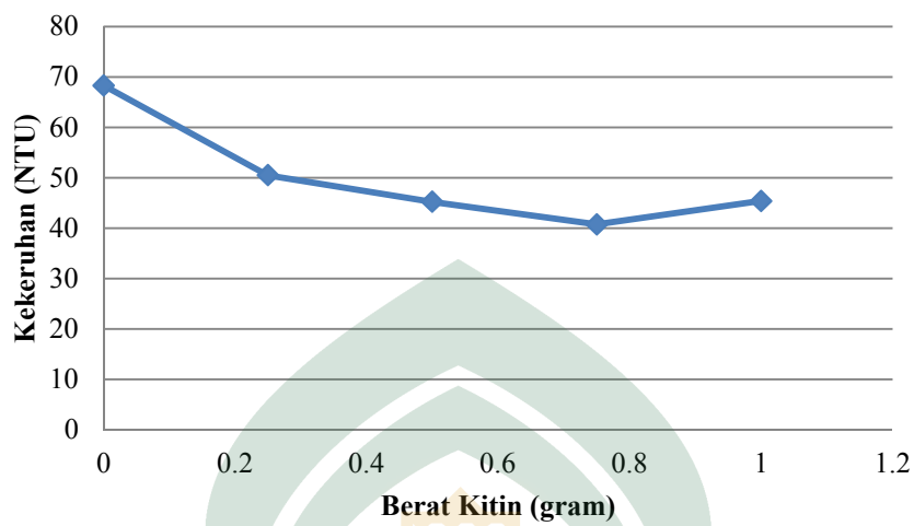
Gambar 4.6 Grafik Hasil Uji Kekeruhan pada Air Sungai setelah Penambahan Kitin
