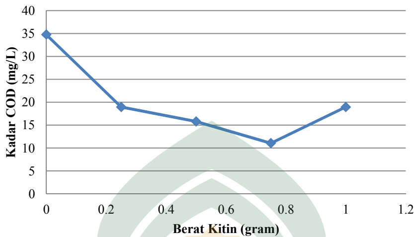
Gambar 4.2 Grafik Hasil Uji COD pada Air Sungai setelah Penambahan Kitin
