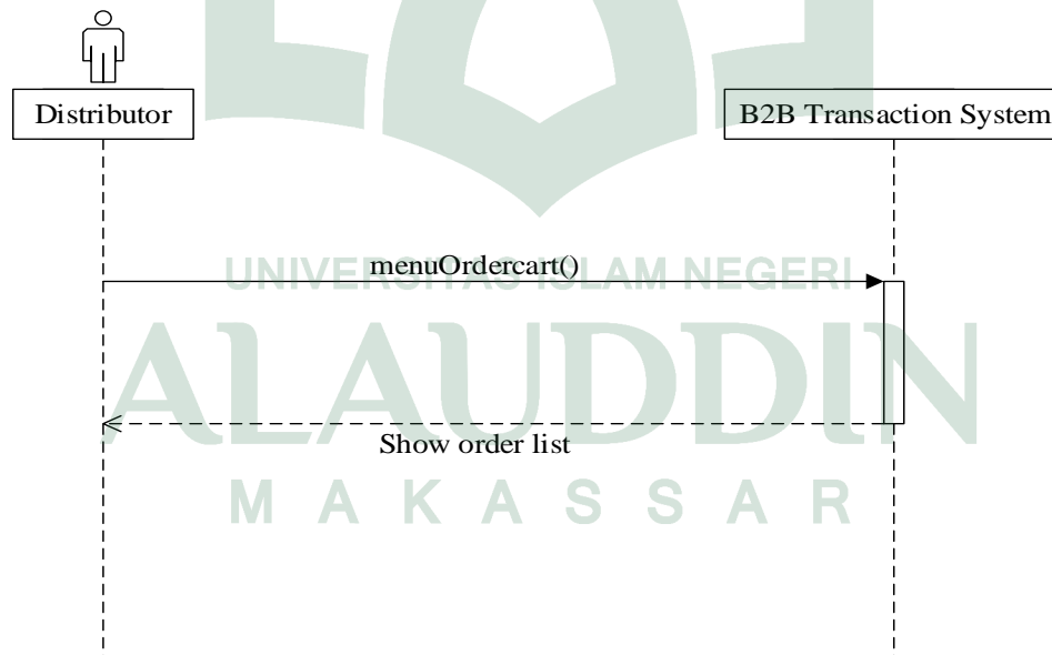
Gambar IV.8 Sequence Diagram untuk melihat Order Cart pada B2B System
