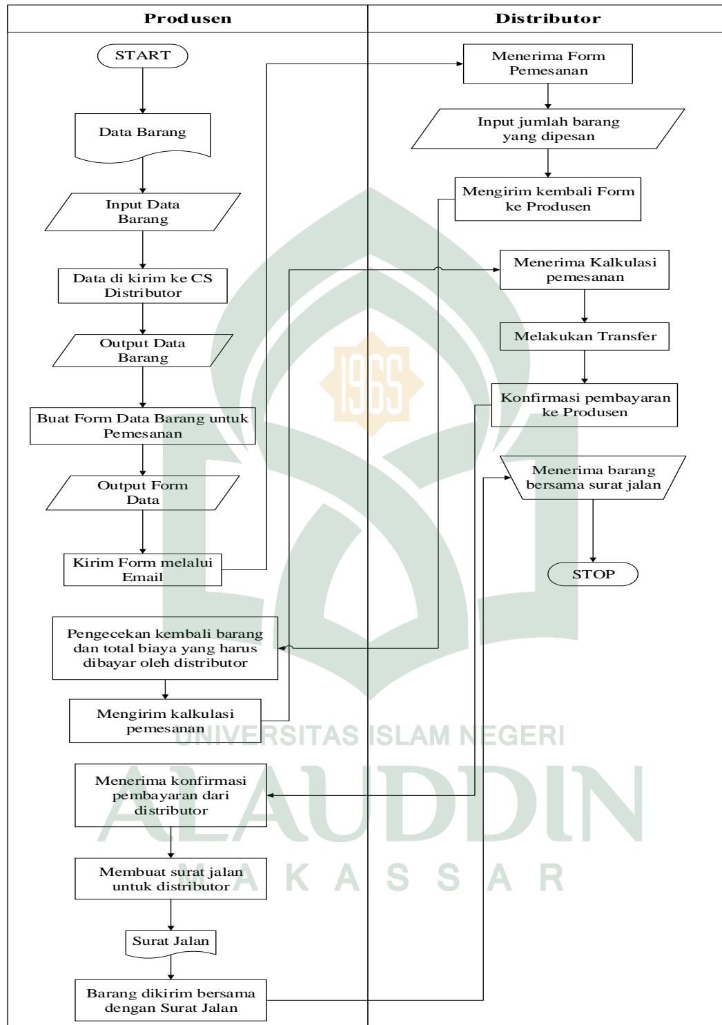
Gambar IV.1 Flowmap Diagram Sistem yang Sedang Berjalan
