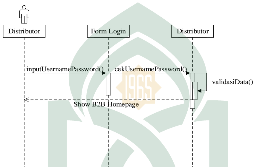
Gambar IV.5 Sequence Diagram untuk Login pada B2B System
