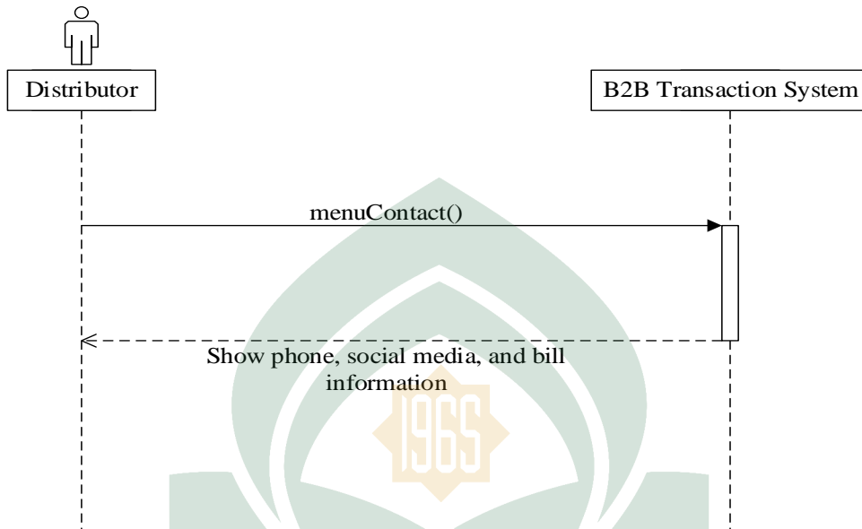
Gambar IV.11 Sequence Diagram untuk melihat Contact us pada B2B System
