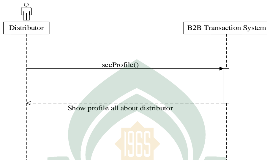
Gambar IV.7 Sequence Diagram untuk melihat Profile pada B2B System
