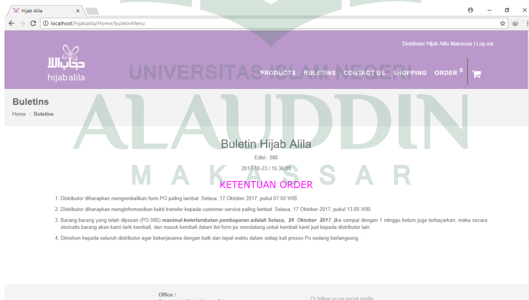
Gambar V.15 Antarmuka Buletin
