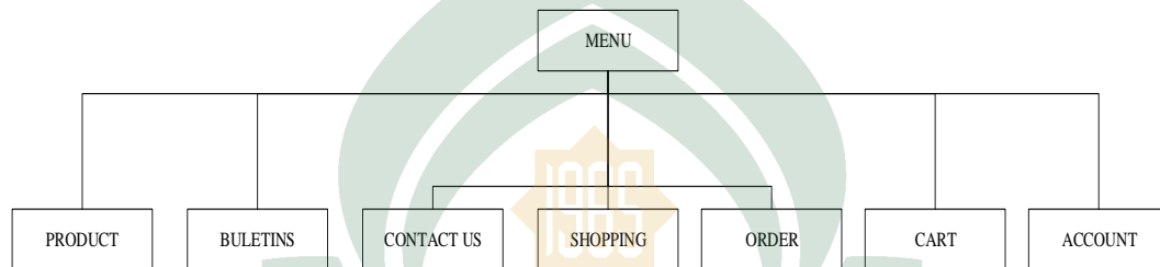
Gambar IV.13 Struktur Navigasi
