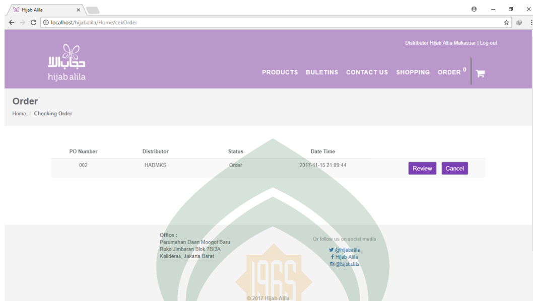
Gambar V.20 Antarmuka Order
