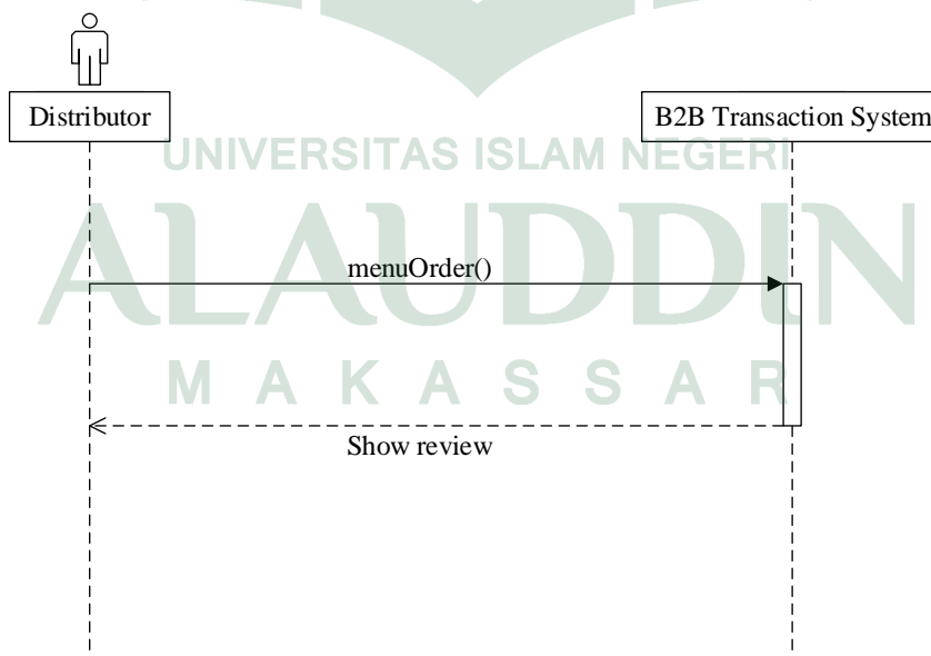
Gambar IV.10 Sequence Diagram untuk melihat Review order pada B2B System
