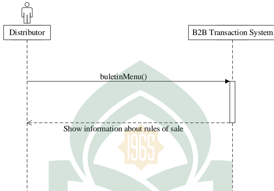
Gambar IV.9 Sequence Diagram untuk melihat Buletin pada B2B System
