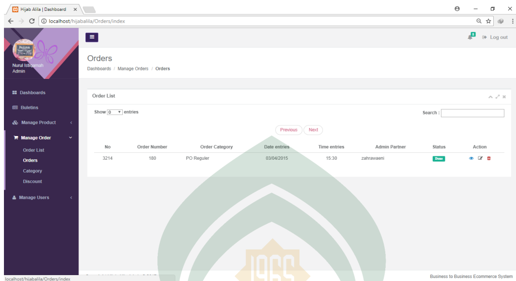
Gambar V.7 Antarmuka Order
