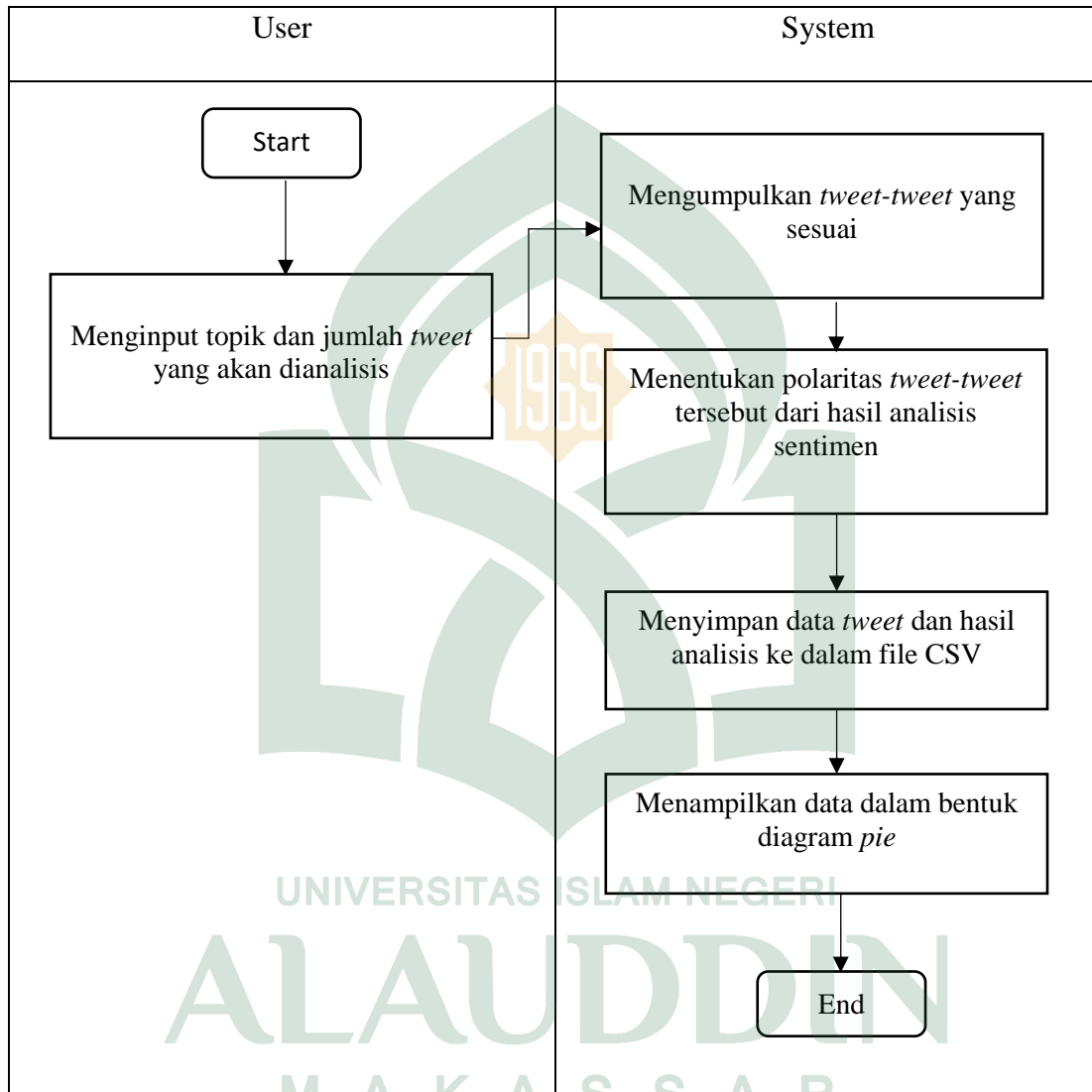
Gambar IV.2 Flowmap pada sistem yang diusulkan
