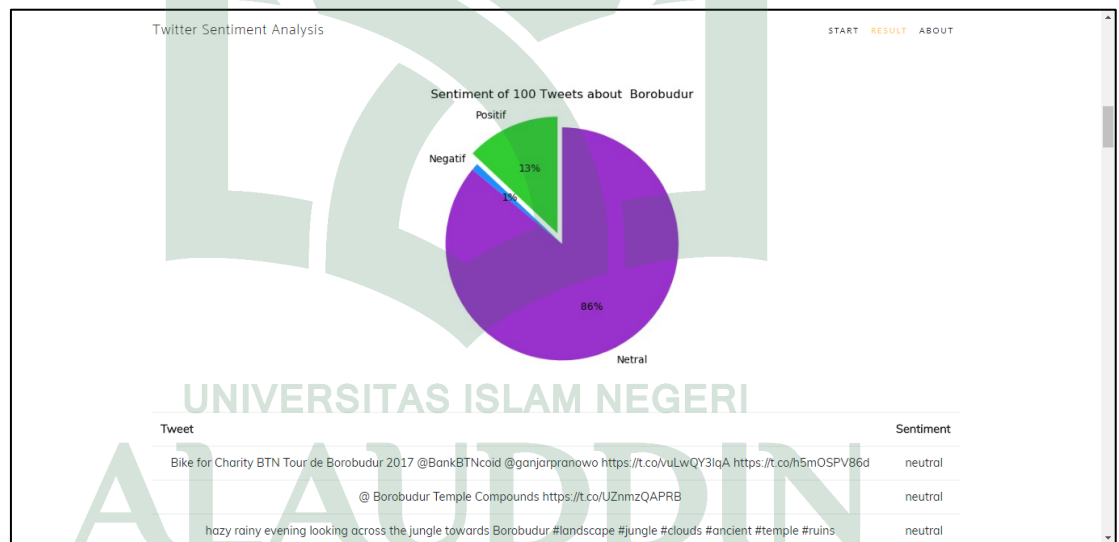
Gambar V.6 Antarmuka Halaman Result pada Topik Borobudur
