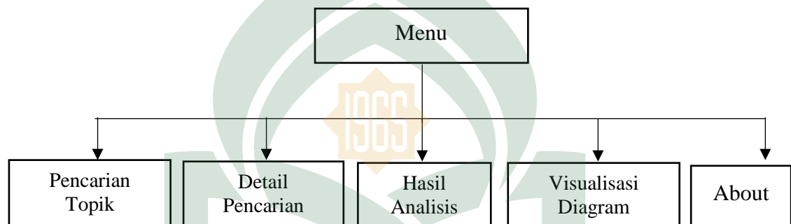
Gambar IV.7 Struktur Navigasi
