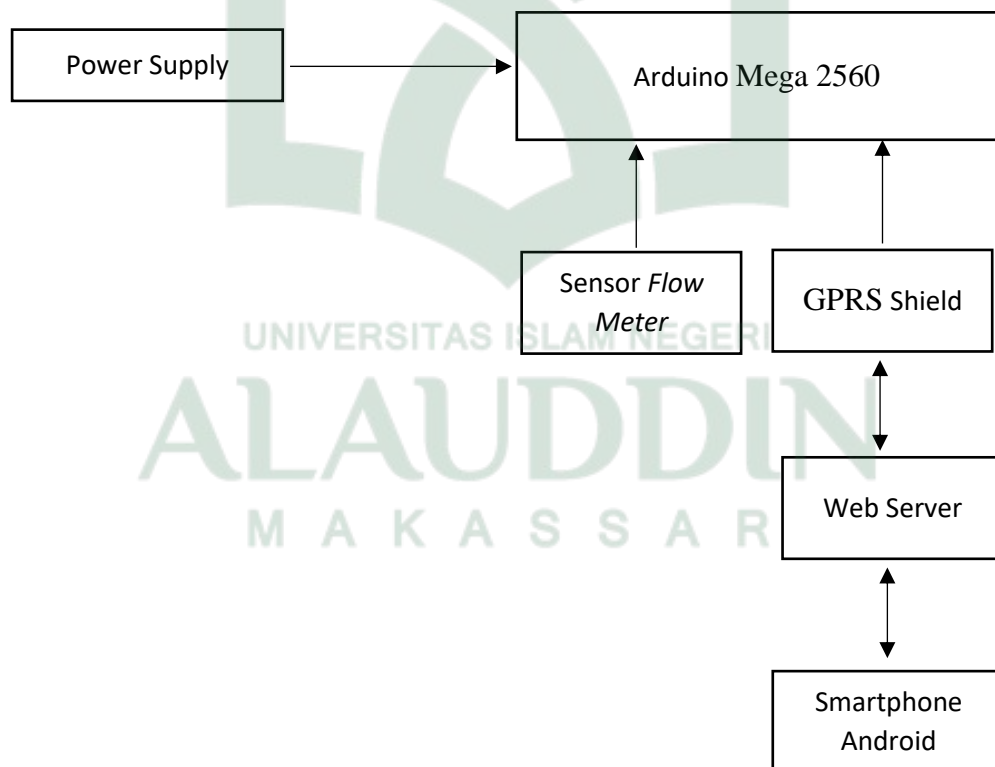
Gambar IV.3 Diagram blok Sistem Pengendalian Penggunaan Air PDAM berbasis Arduino
