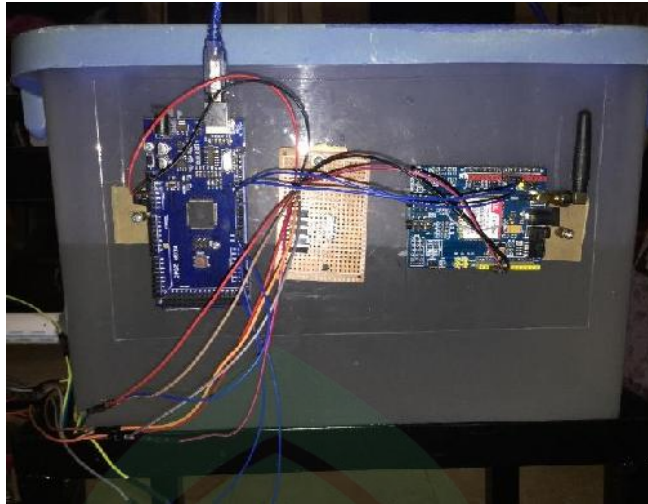
Gambar V.2 Hasil Rancangan Komponen Sistem Pengendalian Penggunaan Air PDAM berbasis Arduino
