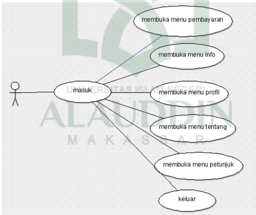
Gambar IV.7 Use Case Diagram Pengguna
