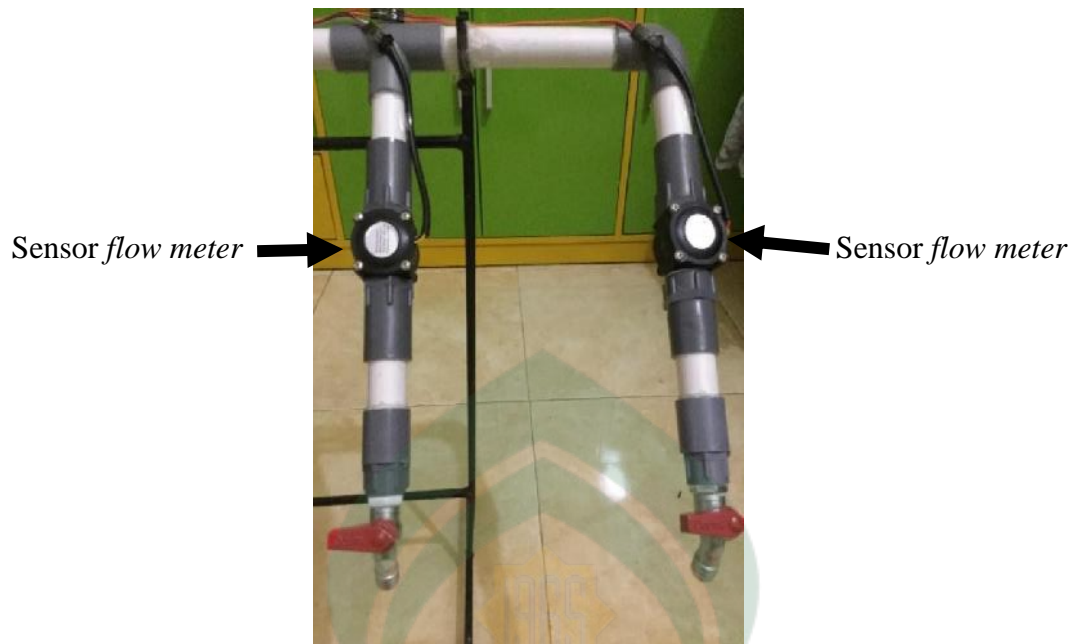
Gambar V.3 Sensor flow meter yang terpasang pada pipa air
