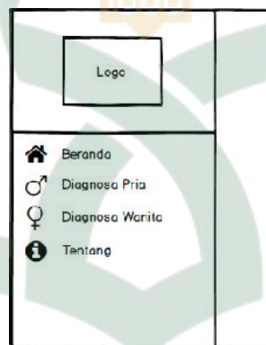
Gambar IV.17 Antarmuka Side Menu
