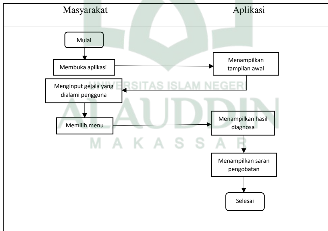
Gambar IV. 2 Flowmap Sistem yang diusulkan
