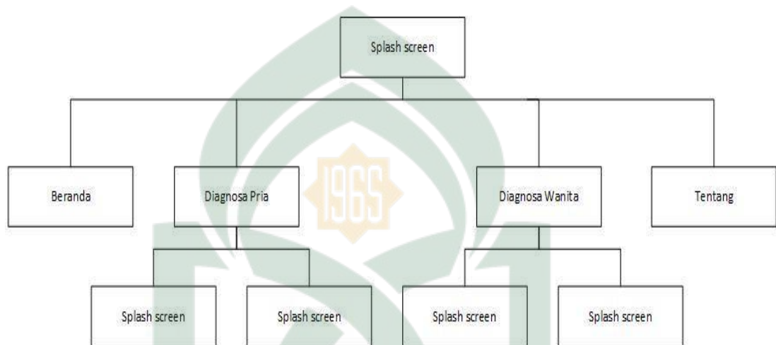
Gambar IV. 8 Struktur Navigasi
