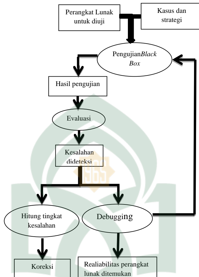
Gambar III.1 Skenario pengujian perangkat lunak terstruktur
