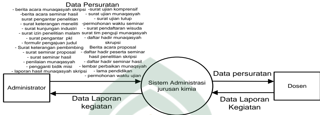
Gambar IV.4 Diagram Konteks
