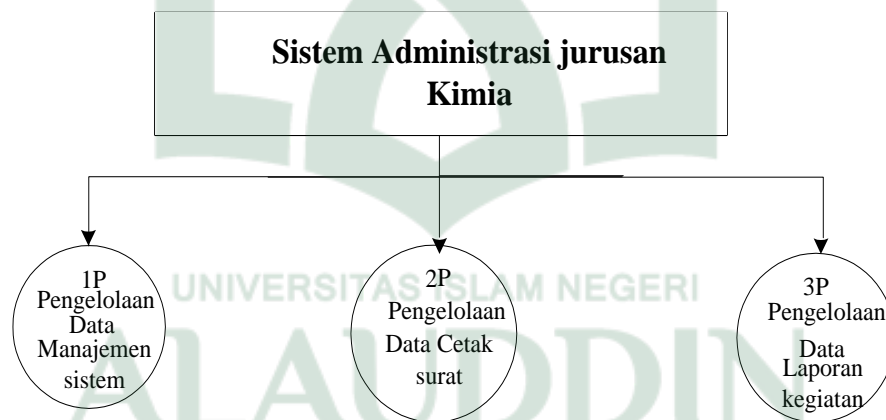
Gambar IV.3 Diagram Berjenjang
