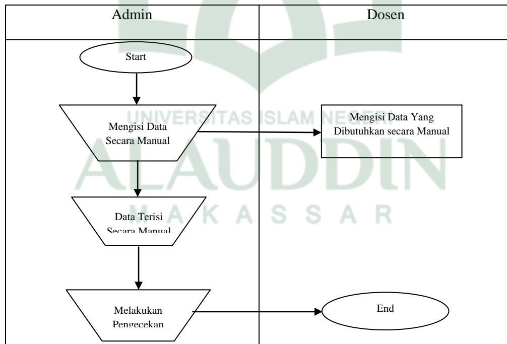
Gambar IV.1 Sistem yang sedang berjalan
