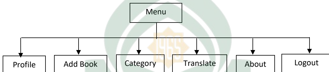
Gambar IV.12 Struktur Navigasi
