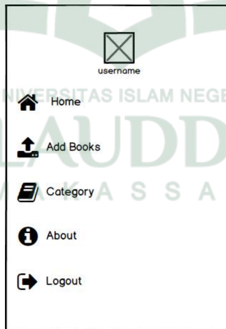
Gambar IV.16 Tampilan Sidebar
