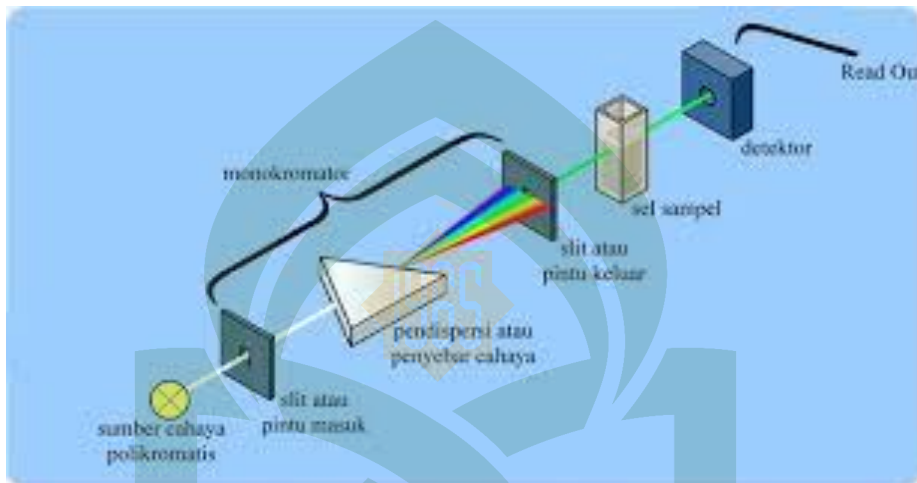
Gambar 2.3. Skema alat spektrofotometer serapan atom
