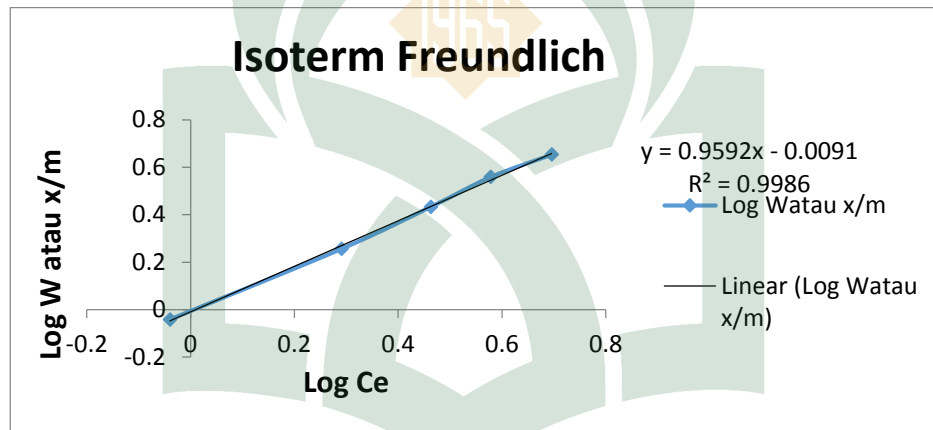
Gambar 4.7. Isoterm Freundlich untuk adsorpsi logam Pb oleh kitin
