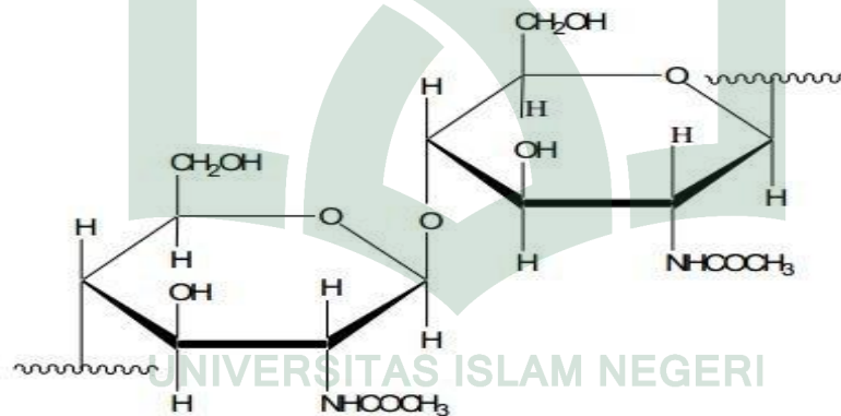
Gambar 2.2. Struktur Konformasi Kitin
