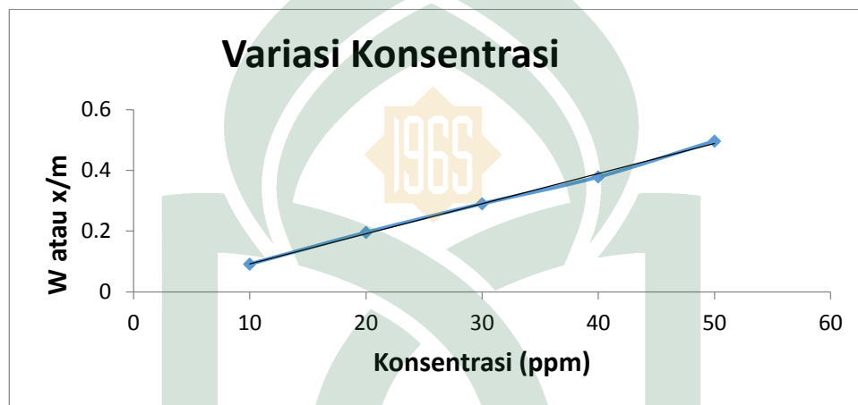
Gambar 4.6. Hubungan antara variasi konsentrasi dan efektivitas adsorpsi (mg/g) kitin terhadap logam Pb dengan waktu kontak 90 menit
