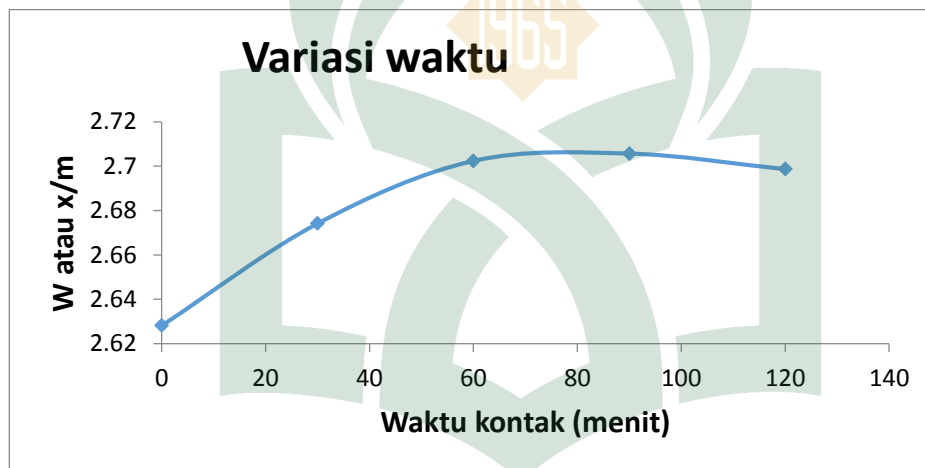
Gambar 4.5. Hubungan antara waktu kontak dan efektivitas adsorpsi (mg/g) kitin terhadap logam Pb dengan konsentrasi 30 ppm
