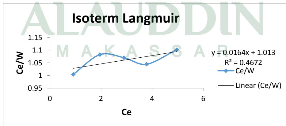
Gambar 4.8. Isoterm Langmuir untuk adsorpsi logam Pb oleh kitin
