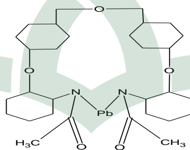
Gambar 4.9. Reaksi kitin dengan logam Pb
