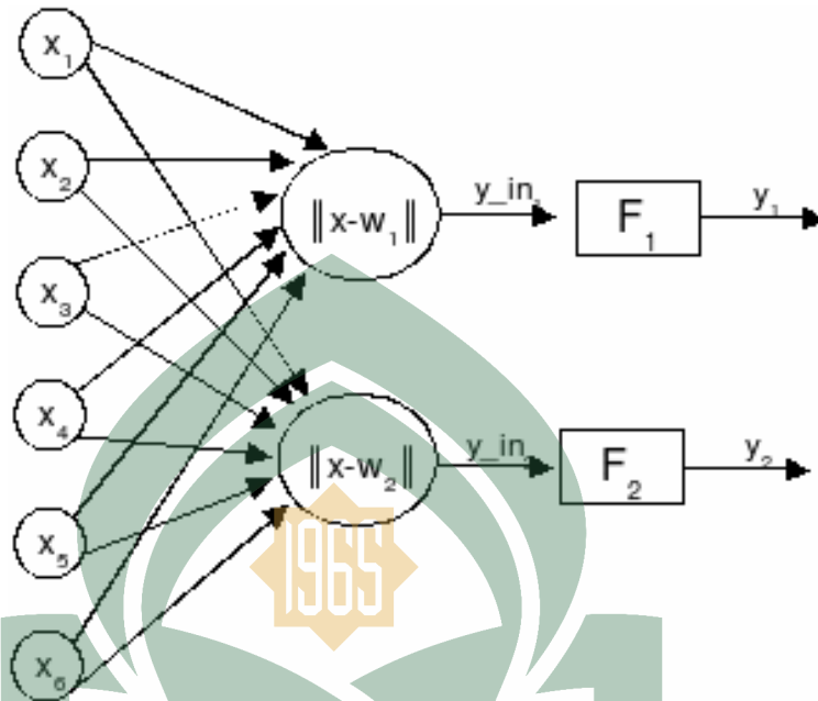
Gambar II.4. Arsitektur Jaringan LVQ.
