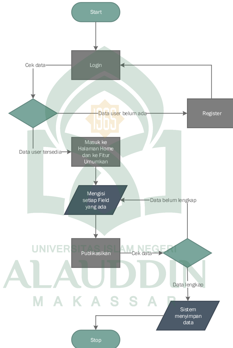
Gambar IV. 24 Flowchart Pengumuman
