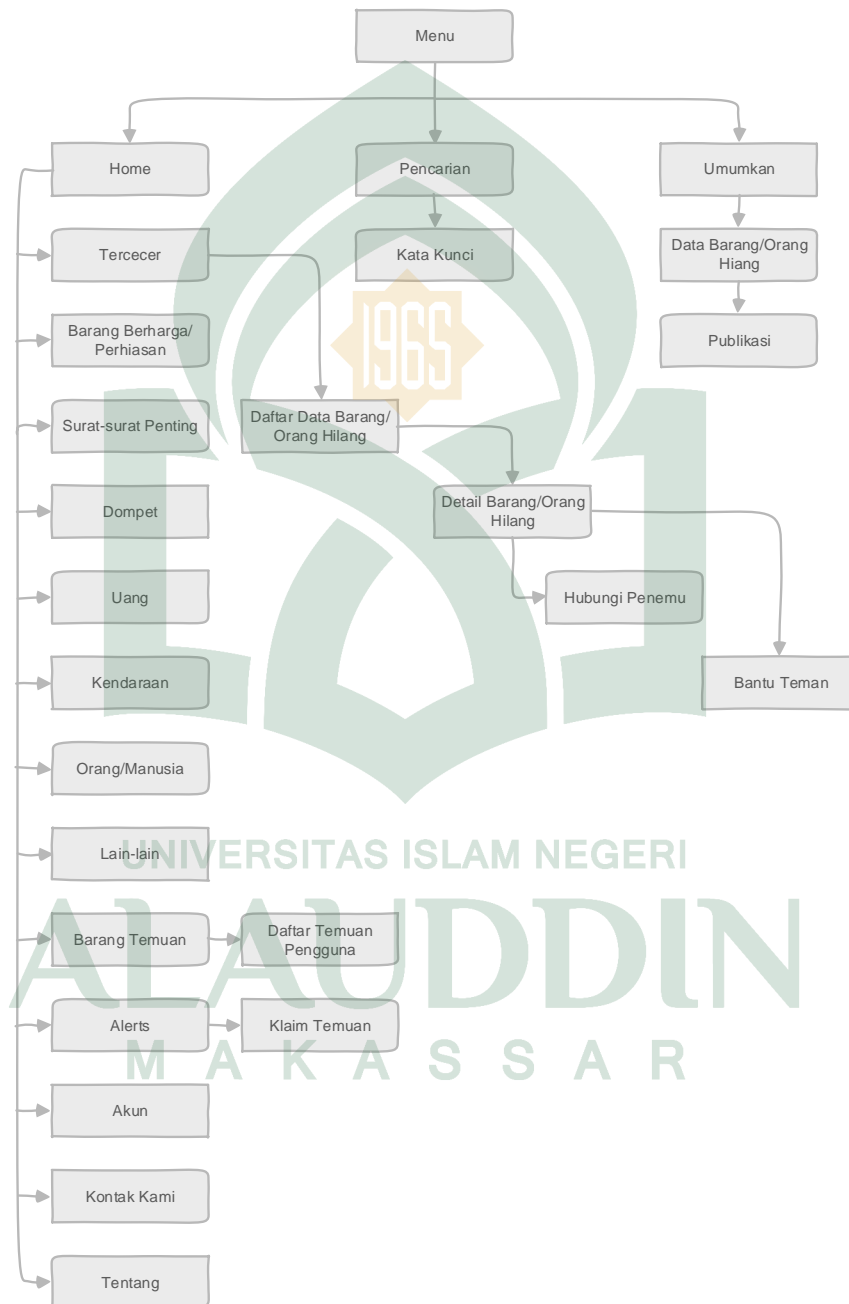
Gambar IV.10 Struktur Navigasi
