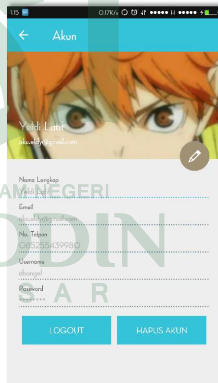
Gambar V.11 Antarmuka Akun
