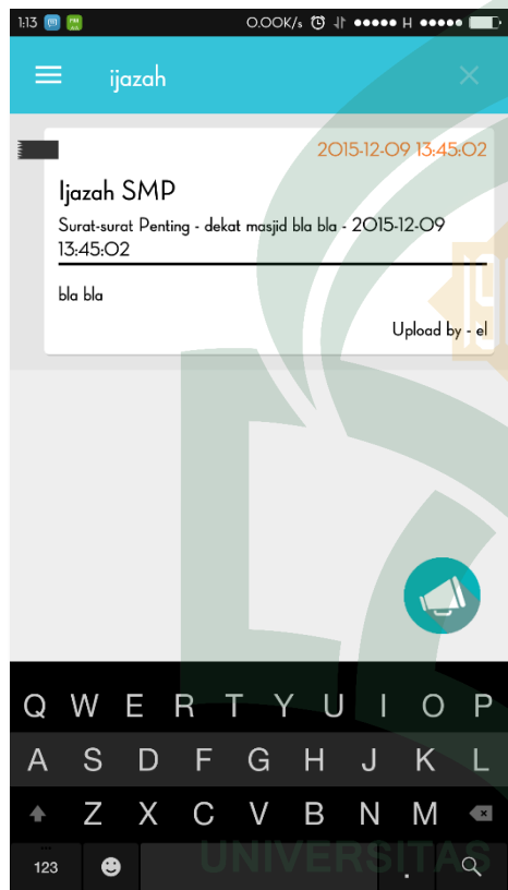
Gambar V.6 Antarmuka Pencarian
