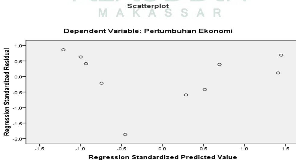
Gambar 4.4 Uji Heteroskedastisitas
