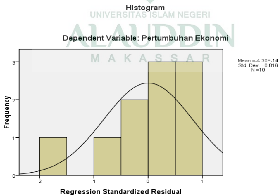
Gambar 4.2 Grafik Histogram
