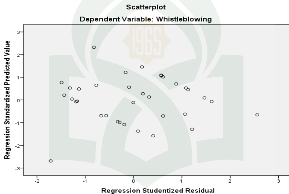
Gambar 4.3 Hasil uji heteroskedastisitas grafik scatterplot
