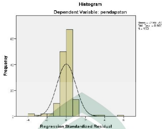
Gambar 4.10 Grafik Histogram
