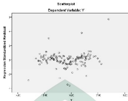
Gambar 4.12 Uji Heteroksedastisitas
