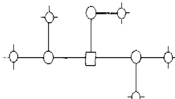
Gambar 2.25 Sistem Jaringan Radial
