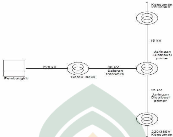
Gambar 2.24 Blok Penyaluran Energi Listrik
