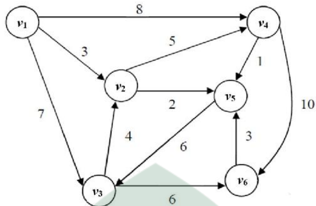
Gambar 2.12 Graf berarah dan berbobot
