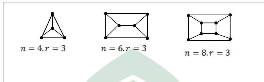
Gambar 2.6 Graf Teratur
