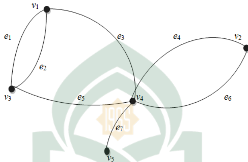
Gambar 2.2 Multigraf
