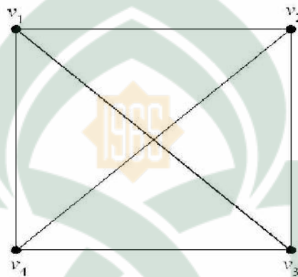
Gambar 2.5 Graf Lengkap
