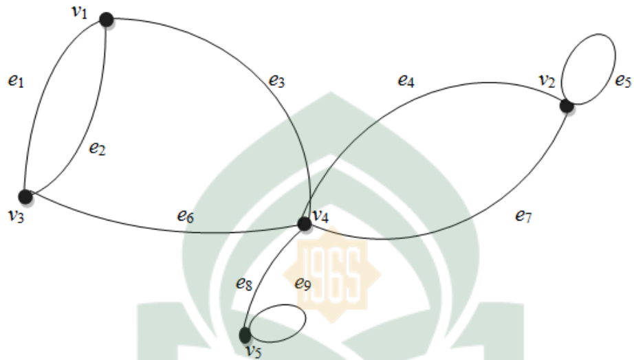
Gambar 2.3 pseudograf
