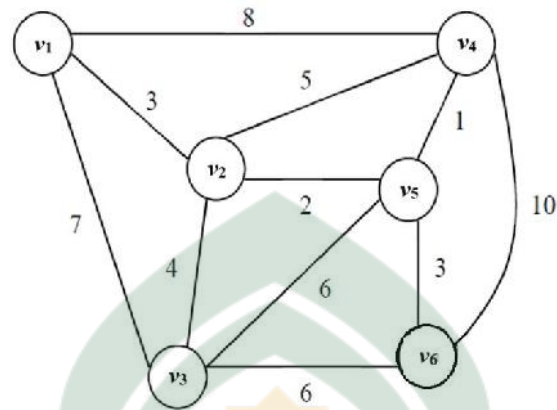
Gambar 2.11 Graf Tak Berarah dan Berbobot
