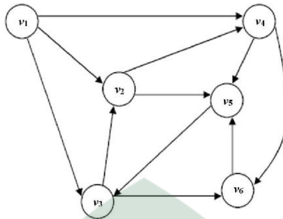
Gambar 2.14 Graf berarah dan tidak berbobot
