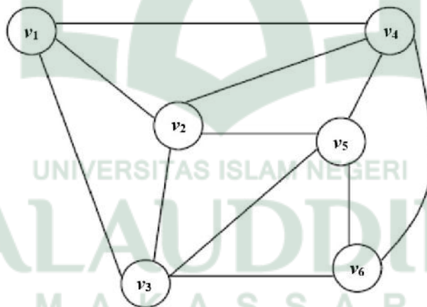
Gambar 2.13 Graf tidak berarah dan tidak berbobot
