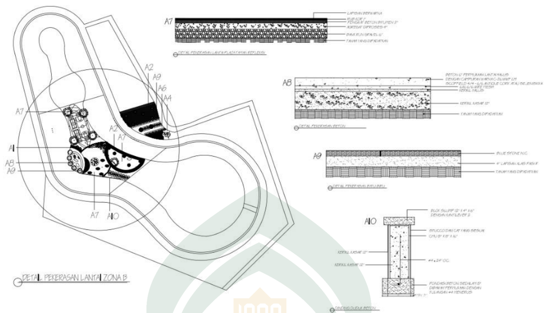
Gambar VI.7 Gambar Pekerasan Lantai Zona B (Sumber: Olah Desain, 2016)
