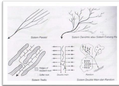
Gambar II.11 Saluran air dalam tanah Sumber : Hakim,Rustam 2012:280
