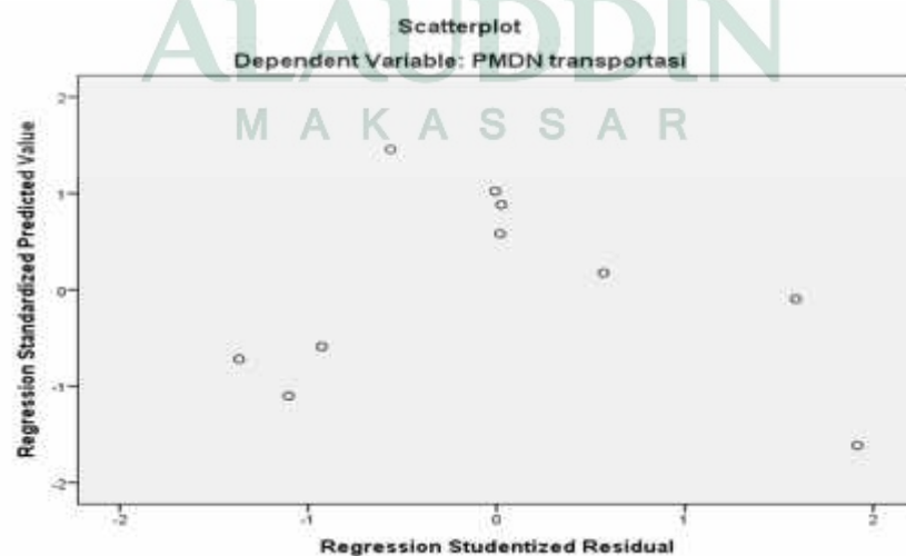
Gambar 4.3 Uji Heterokedastisitas
