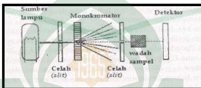
Gambar 2.5 Skema instrument UV-Vis Sumber: http://www.google.co.id
