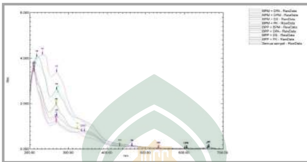
Gambar 4.21 Grafik penggabungan semua data grafik
