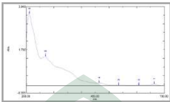
Gambar 4.7 Grafik hasil uji UV-Vis ekstrak bunga pacar merah dan daun putri malu sesudah pencampuran
