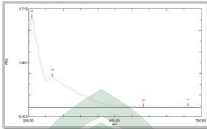
Gambar 4.9 Grafik hasil uji UV-Vis ekstrak bunga pacar merah dan daun sirsak sesudah pencampuran
