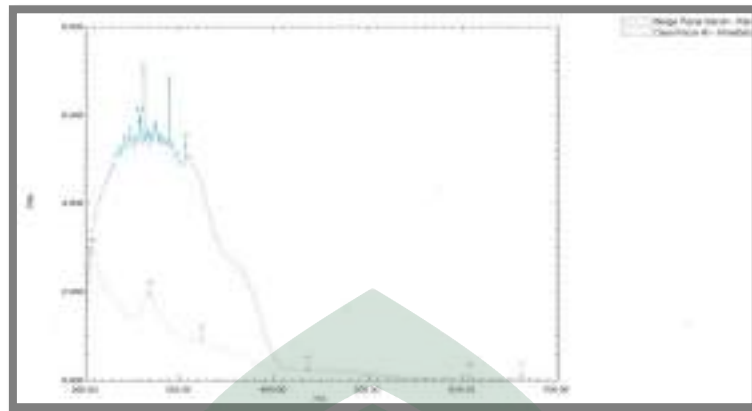
Gambar 4.4 Grafik hasil uji UV-Vis ekstrak bunga pacar merah dan daun pacar air sebelum pencampuran
