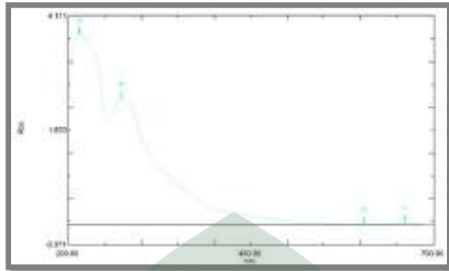
Gambar 4.11 Grafik hasil uji UV-Vis ekstrak bunga pacar merah dan daun pacar kuku sesudah pencampuran
