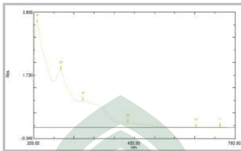
Gambar 4.15 Grafik hasil uji UV-Vis ekstrak bunga pacar putih dan daun pacar air sesudah pencampuran
