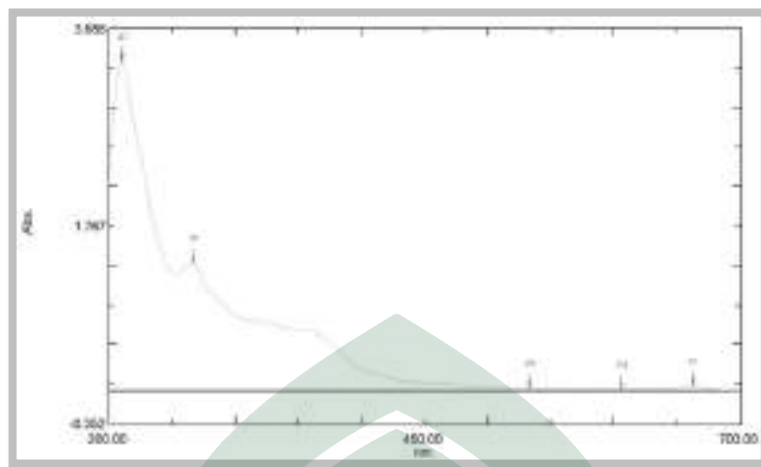
Gambar 4.17 Grafik hasil uji UV-Vis ekstrak bunga pacar putih dan daun sirsak sesudah pencampuran
