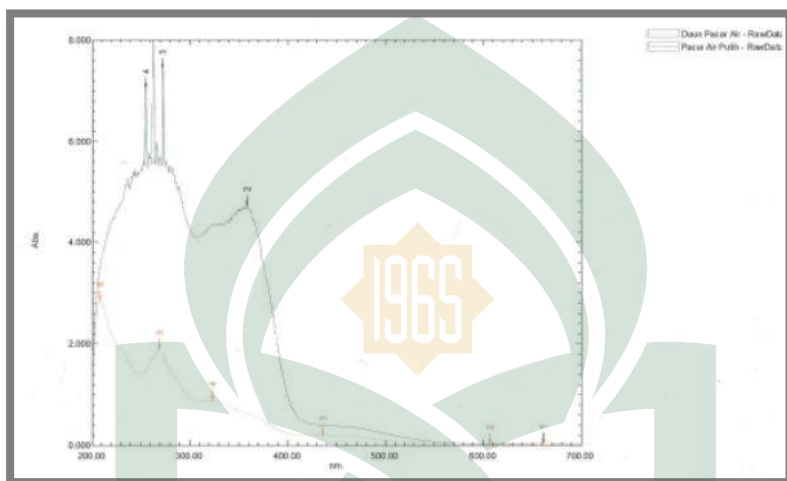
Gambar 4.14 Grafik hasil uji UV-Vis ekstrak bunga pacar putih dan daun pacar air sebelum pencampuran
