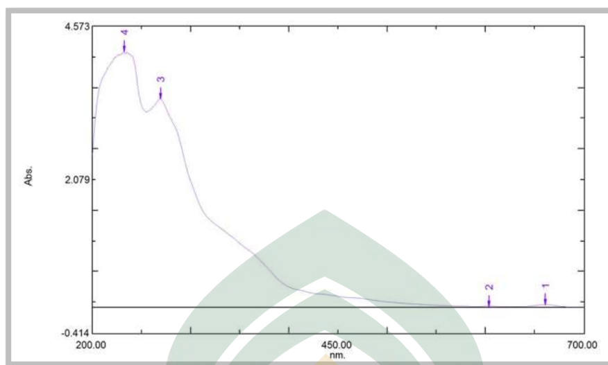
Gambar 4.19 Grafik hasil uji UV-Vis ekstrak bunga pacar putih dan daun pacar kuku sesudah pencampuran
