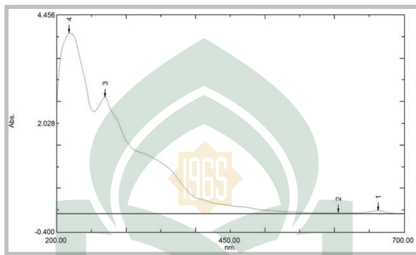
Gambar 4.20 Grafik hasil uji UV-Vis ekstrak Semua Sampel
