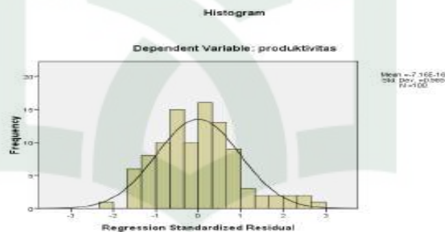
Gambar 4.1 : Grafik Histogram
