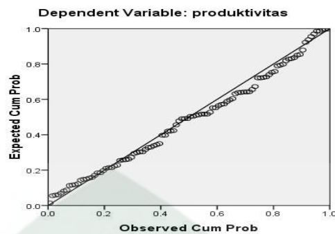
Gambar 4.2 : grafik Normal P-Plot
