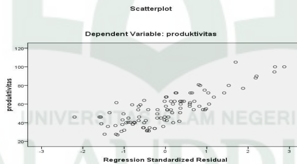
Gambar 4.4 : Uji Heterokedastisitas
