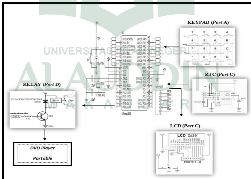
Gambar IV.8 Rangkaian Keseluruhan
