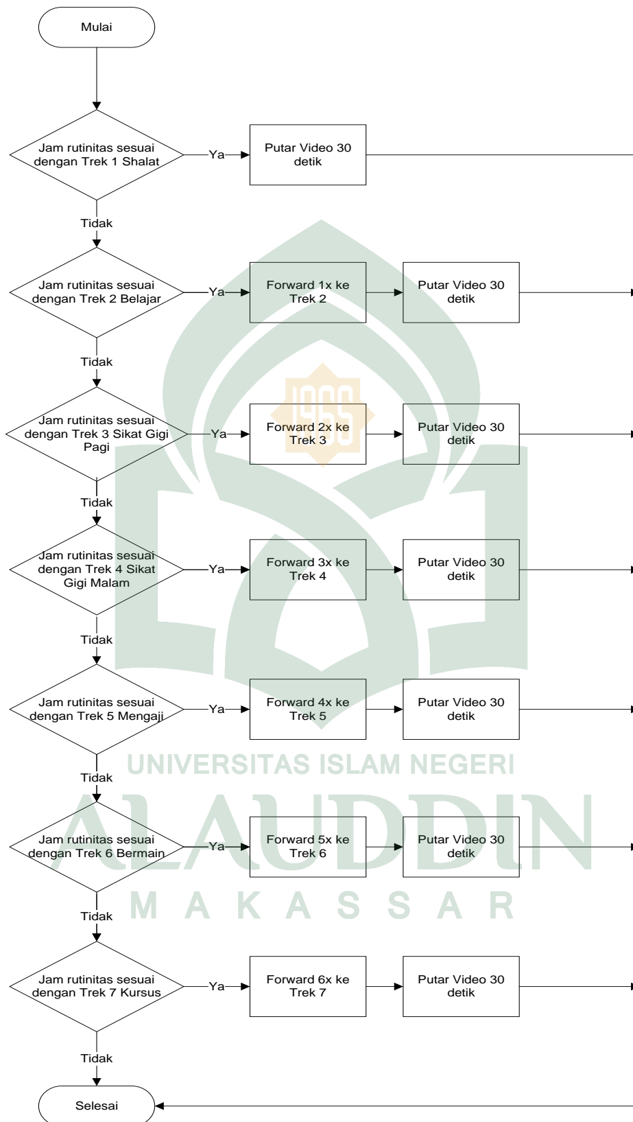
Gambar III.1 Tahapan Pengujian Alat dengan Metode Blackbox
