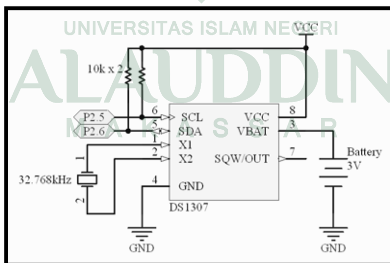
Gambar IV.4 Rangkaian RTC (Sumber : www.tronixstuff.com , 2014)
