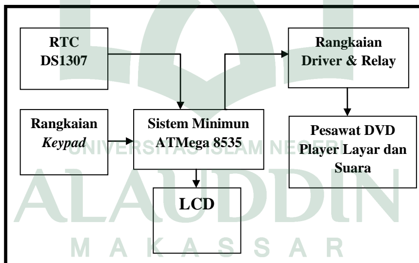
Gambar IV.2 Blok Diagram Rancangan Sistem Secara Umum
