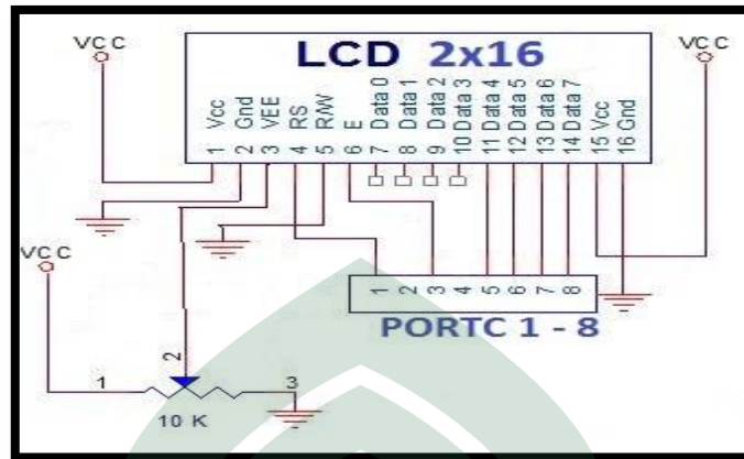
Gambar IV.5 Rangkaian LCD (Sumber : www.etekno.blogspot.com , 2014)
