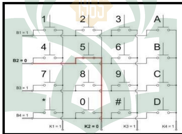
Gambar IV.6 Teknik Pembacaan ( Scanning ) Keypad 4×4
