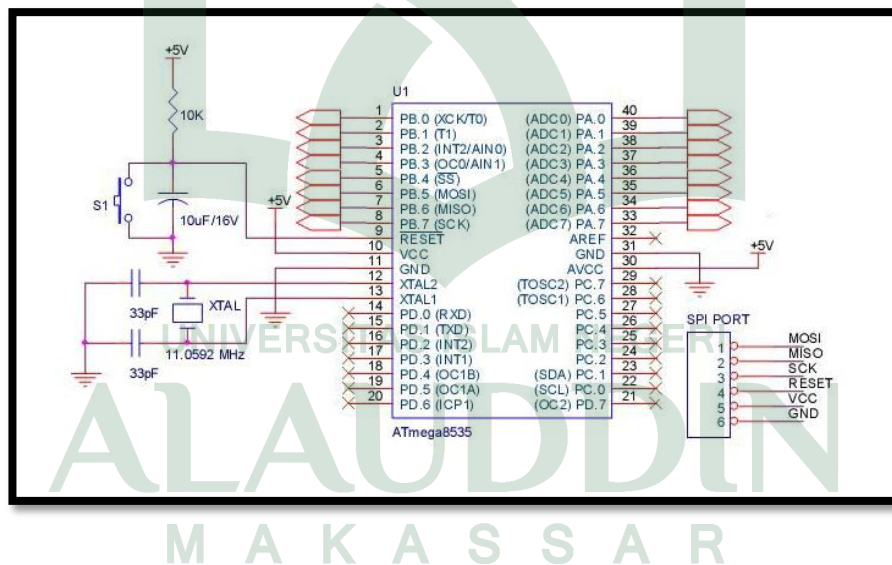
Gambar IV.3 Rangkaian Sistem Minimum Mikrokontroler Atmega 8538
