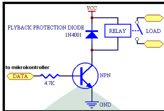
Gambar IV.7 Rangkaian Relay (Sumber : Wikipedia, 2014)
