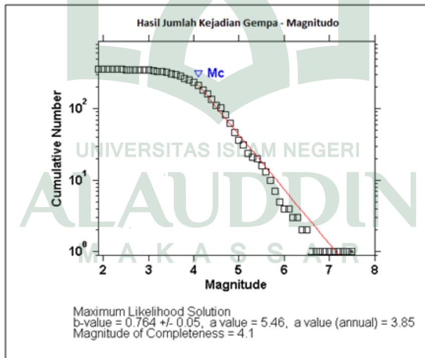
Gambar 4.4: Grafik hubungan antara frekuensi dan magnitudo
