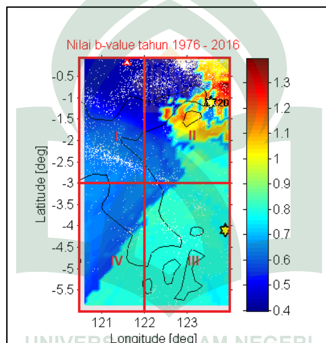
Gambar 4.7: Perbandingan sebaran nilai b-value setelah dibagi menjadi 4 kwartal
