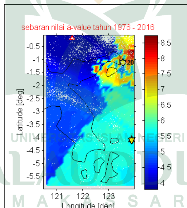
Gambar 4.8: Sebaran nilai a-value sebelum dibagi menjadi 4 kwartal
