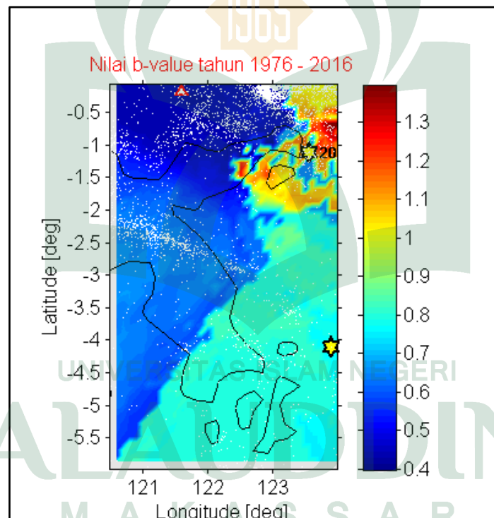
Gambar 4.6: Sebaran nilai b -value sebelum dibagi menjadi 4 kwartal
