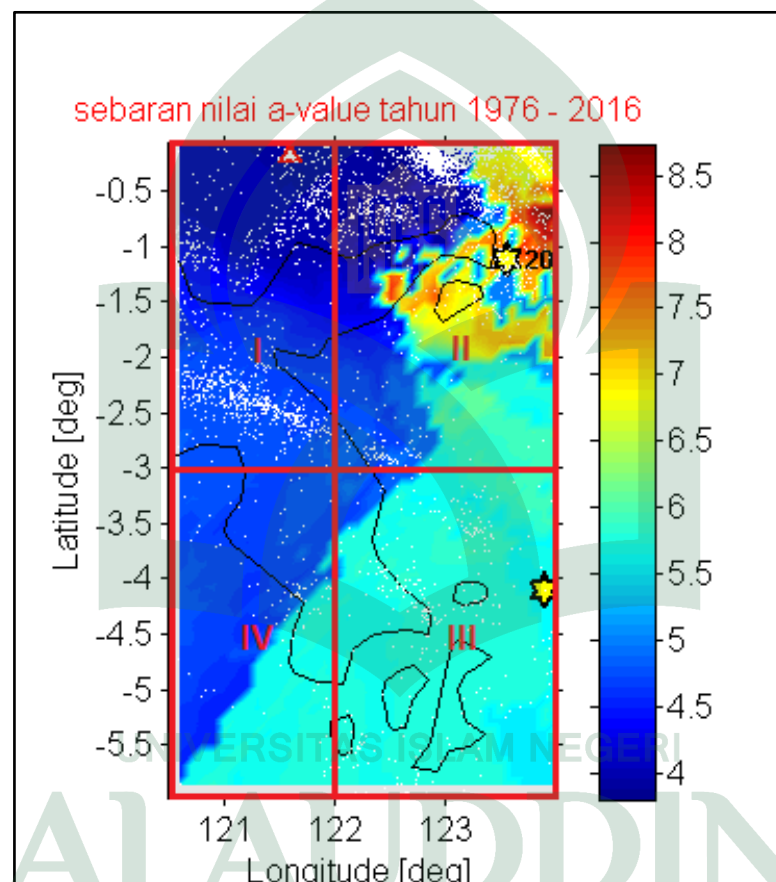
Gambar 4.9: Perbandingan nilai sebaran a – value setelah dibagi menjadi 4 kuartal
