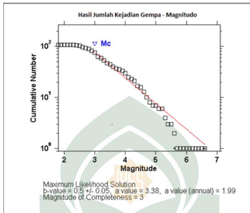
Gambar 4.5: Grafik hubungan antara frekuensi dan magnitudo
