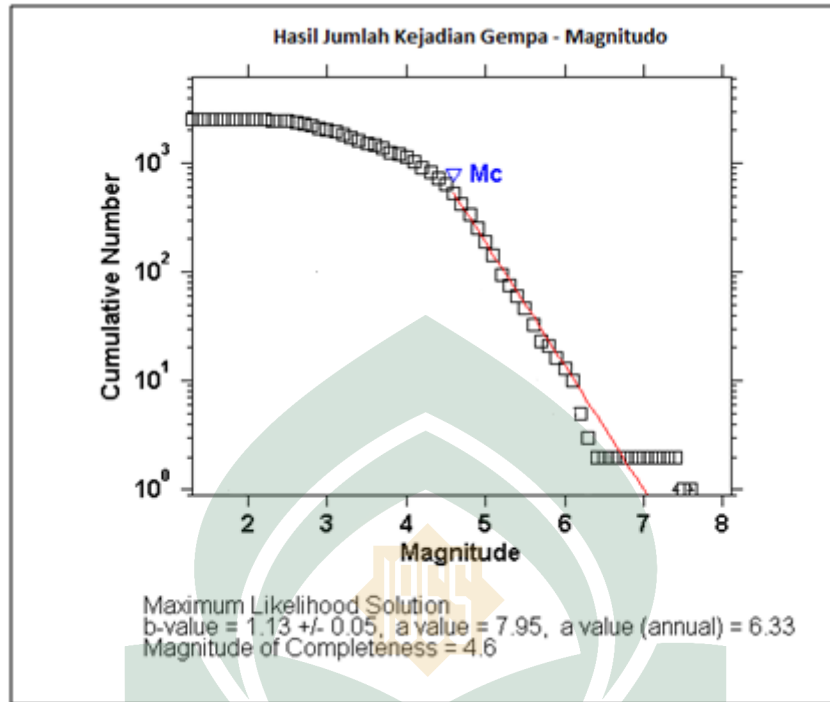
Gambar 4.3: Grafik hubungan antara frekuensi dan magnitudo
