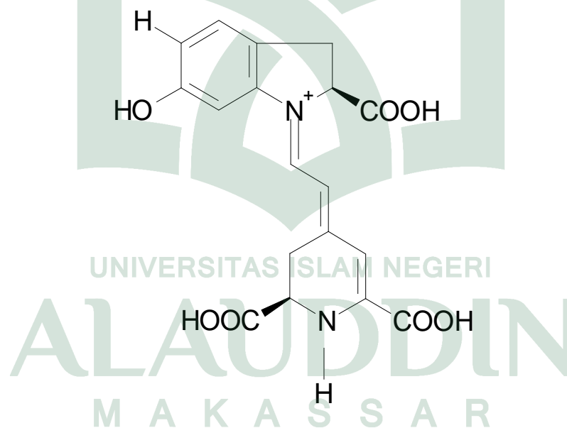
Gambar 2.5. Struktur Betasianin
