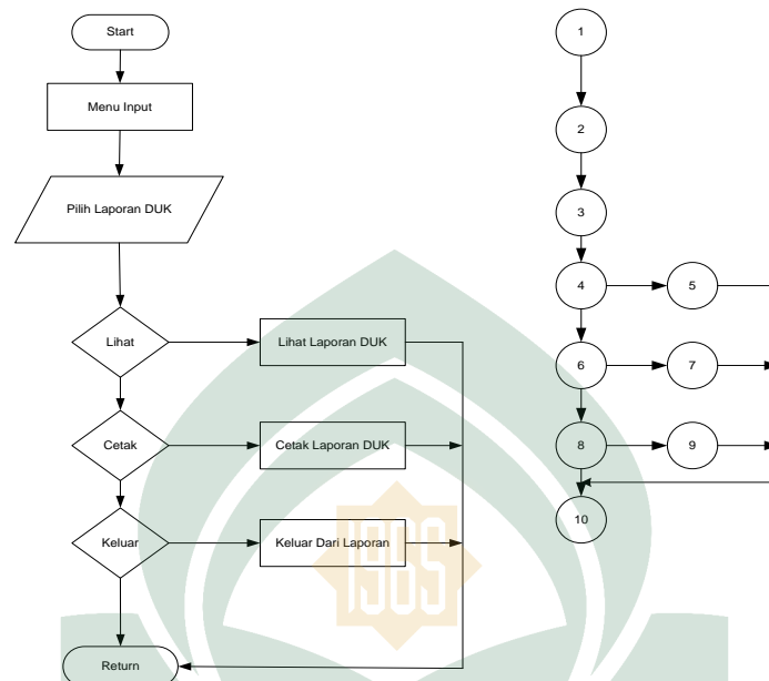
Gambar V.8 Flowchart dan Flowgraph Form Laporan Daftar Urut Kepangkatan
