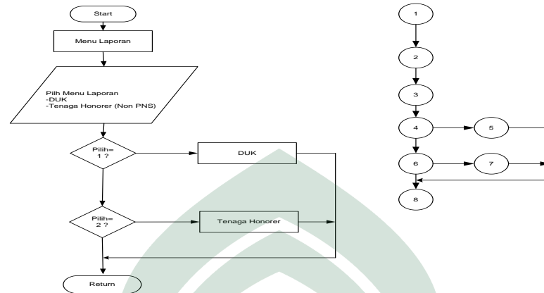
Gambar V.2 Flowchart dan Flowgraph Menu Laporan
