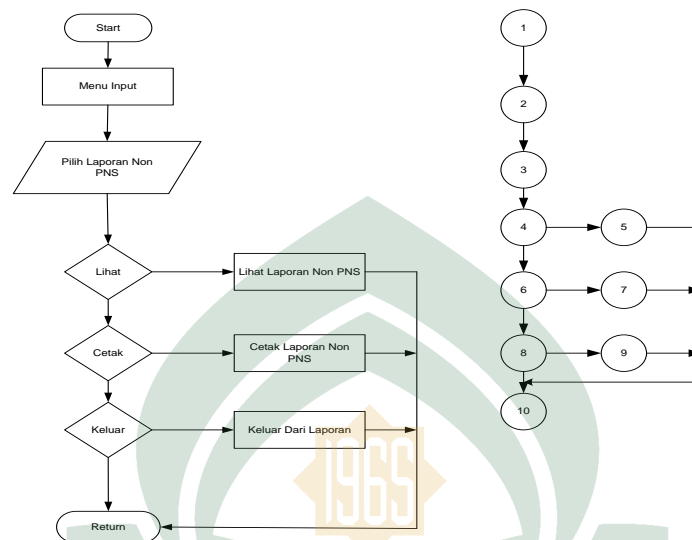
Gambar V.9 Flowchart dan Flowgraph Form Laporan Daftar Tenaga Honorer
