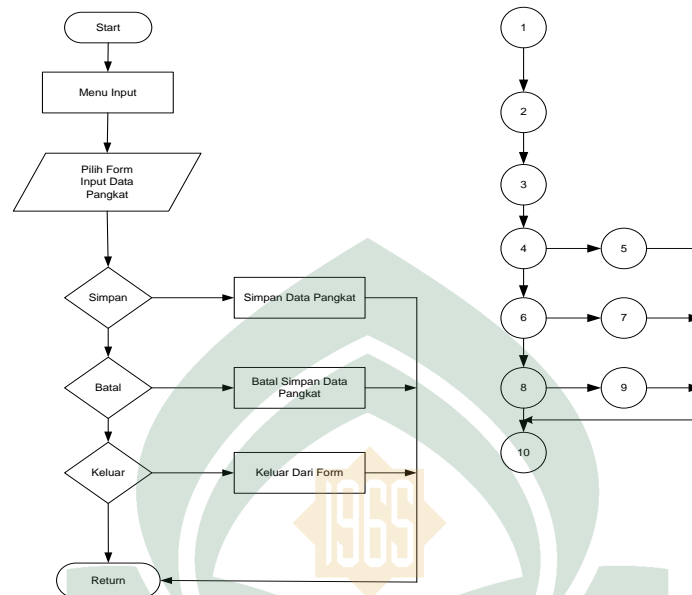
Gambar V.6 Flowchart dan Flowgraph Form Input Data Pangkat
