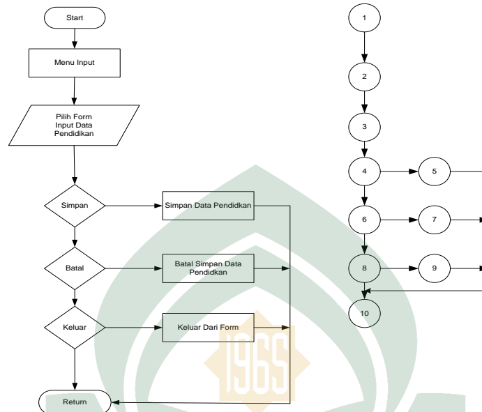
Gambar V. 4 Flowchart dan Flowgraph Form Menu Input Data Pendidikan
