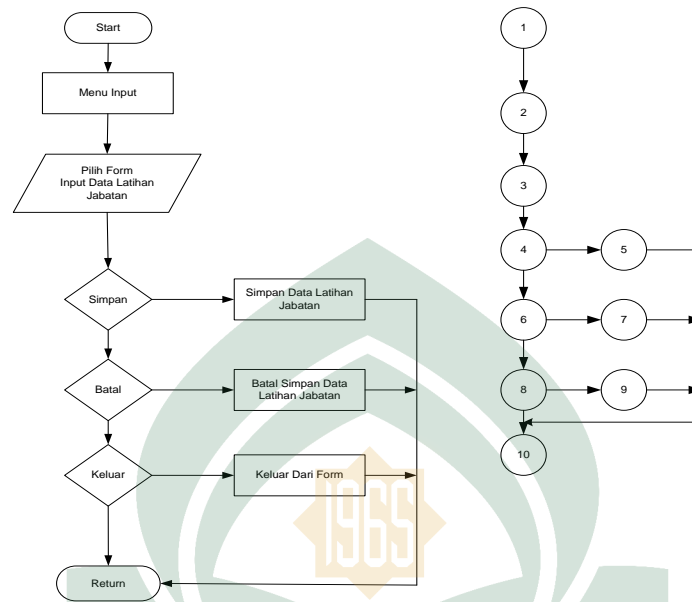
Gambar V.7 Flowchart dan Flowgraph Form Input Data Latihan Jabatan
