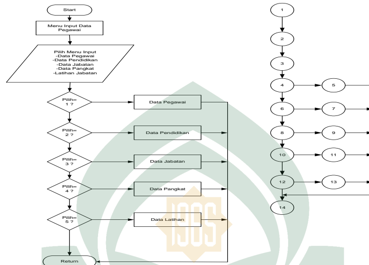
Gambar V.1 Flowchart dan Flowgraph Menu Input Data
