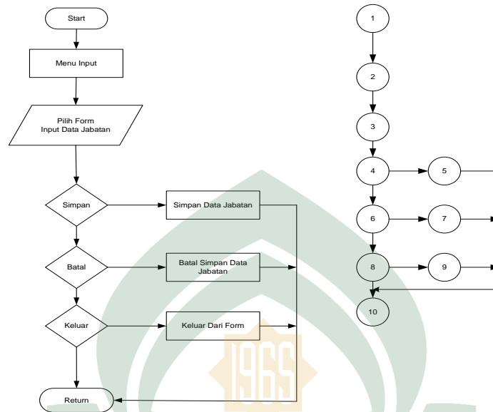
Gambar V.5 Flowchart dan Flowgraph Form Input Data Jabatan
