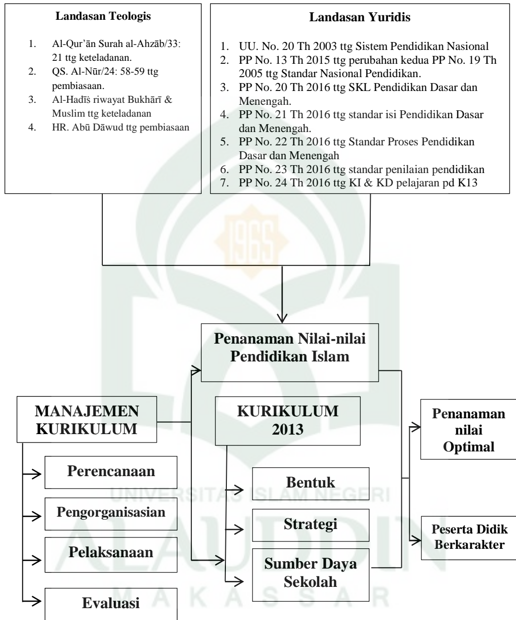
Gambar 2.2 Kerangka Konseptual
