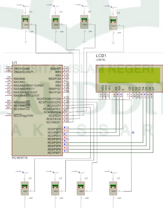
Gambar IV.7 Rangkaian Simulasi Modul Alat Sistem Perparkiran
