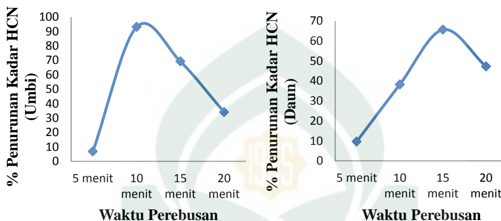
Gambar 4.5. Kurva Penentuan waktu optimum perebusan pada umbi dan daun
