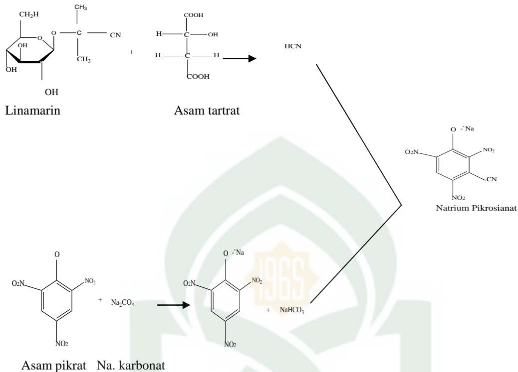
Gambar 4.1. Reaksi pembentukan Natrium Pikosianat
