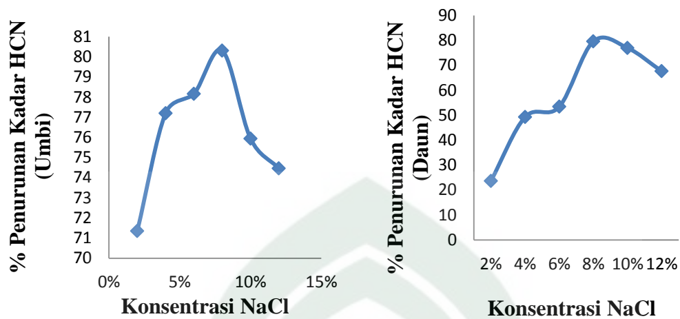
Gambar 4.4. Kurva Penentuan Konsentrasi optimum NaCl pada umbi dan daun
