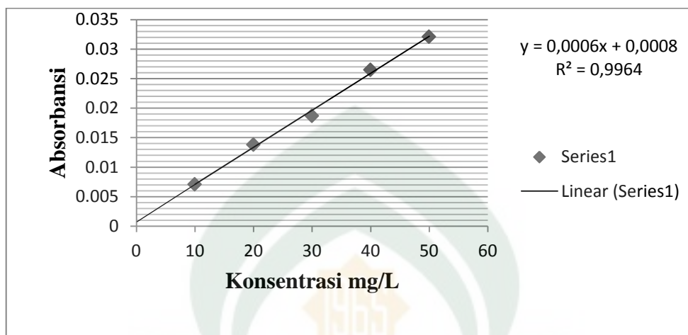
Gambar 6.1 Hubungan antara Absorbansi dan Konsentrasi Standar
