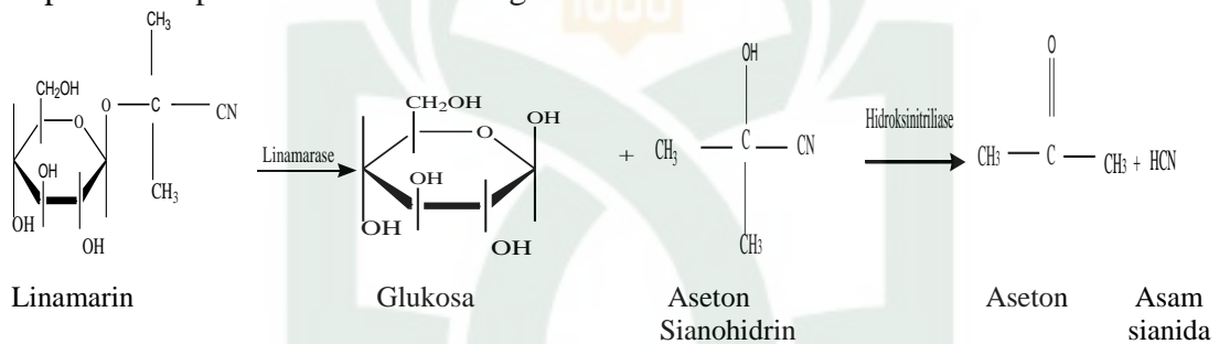
Gambar 4.2. Reaksi Pembentukan Asam Sianida (HCN)
