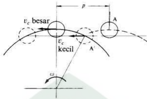
Gambar II.6 Variasi kecepatan rantai rol
