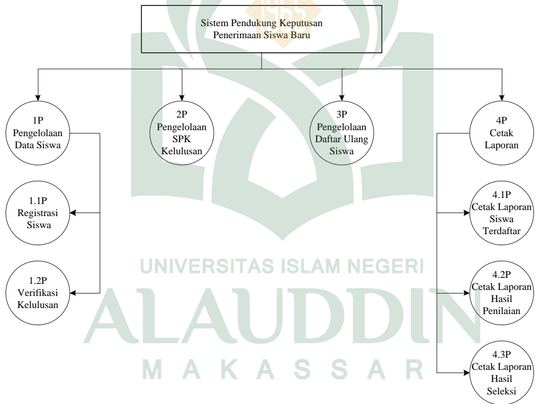
Gambar IV.3 Diagram Berjenjang
