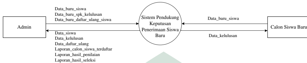
Gambar IV.4 Konteks Diagram
