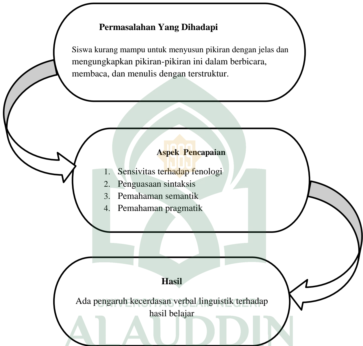
Gambar 4.1 Kerangka Berpikir
