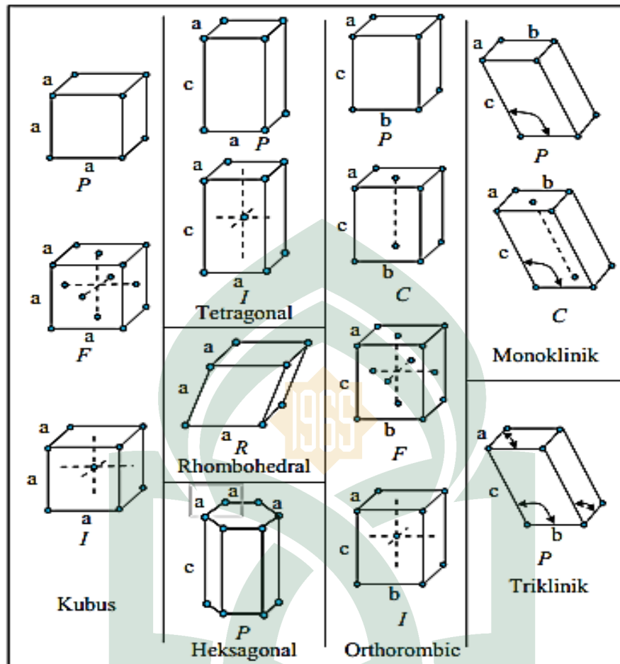
Gambar 2.6. Sel unit dari 14 kisi ruang Bravais (Sumber: Sudaryatmou & Ning, 2010)
