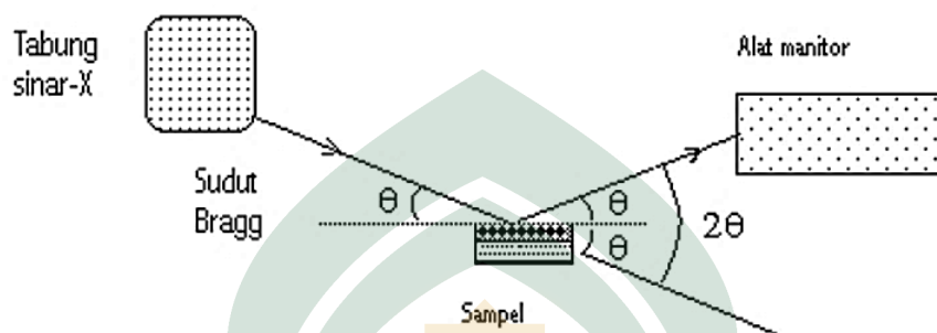
Gambar 2.5. Skema Difraktometer Serbuk (Sumber: Asmuni, 2014)
