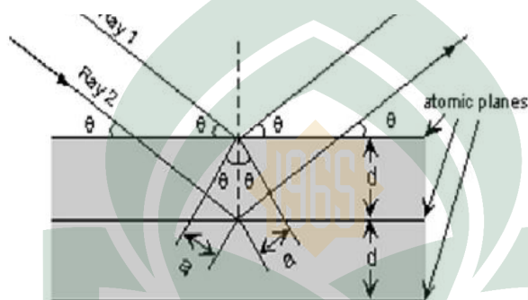
Gambar2.4. Difraksi Sinar X (Sumber: Nelson, 2010).
