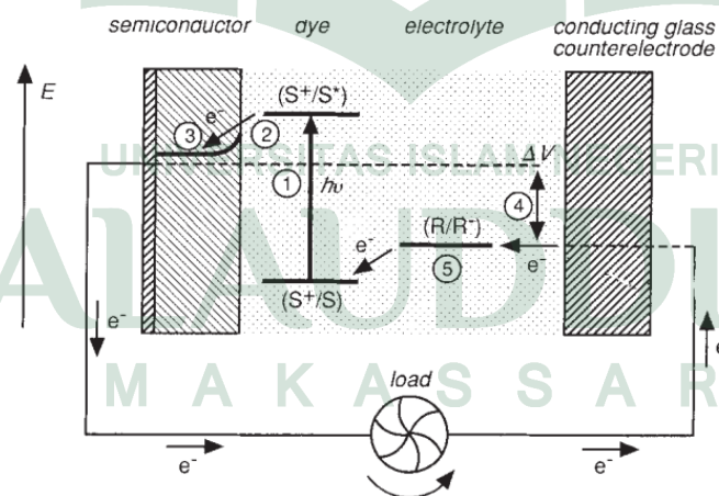
Gambar 2.2. Susunan Satu Sel DSSC (Gartzel dan O'regan, 1991: 2).
