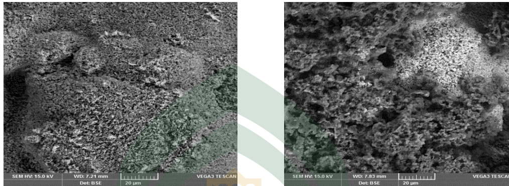
Gambar 4.1 (a) Morfologi \text{TiO}_2 20 \mu\text{m} (b) Morfologi \text{TiO}_2 terikat dengan dye dari daun jati (20 \mu\text{m} )
