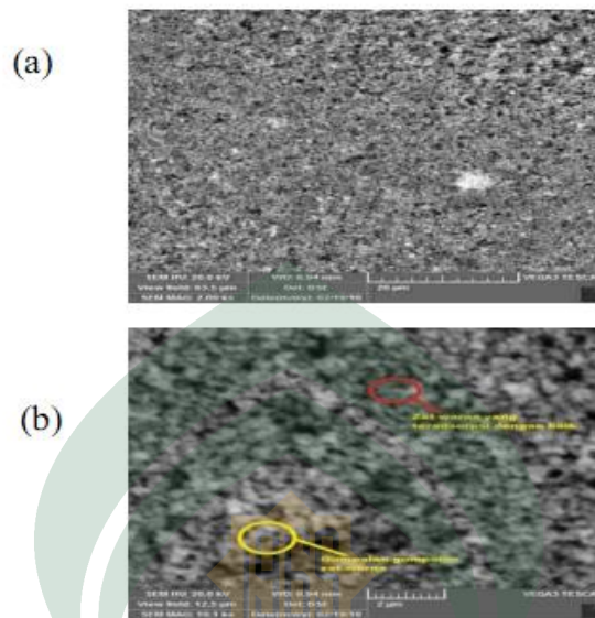
Gambar 2.8. Hasil SEM permukaan TiO 2 yang mengikat zat warna a.20 μm dan b. 2 μm
