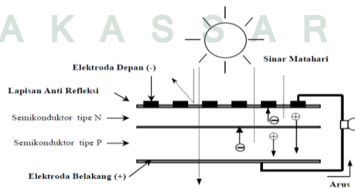
Gambar 2.1. Proses Pengubahan Energi Matahari Menjadi Energi Listrik
