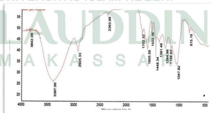
Gambar 4.6. Hasil serapan FTIR Ekstrak Metanol Daun Jati
