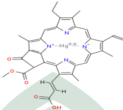
Gambar 2.6. Struktur Klorofil
