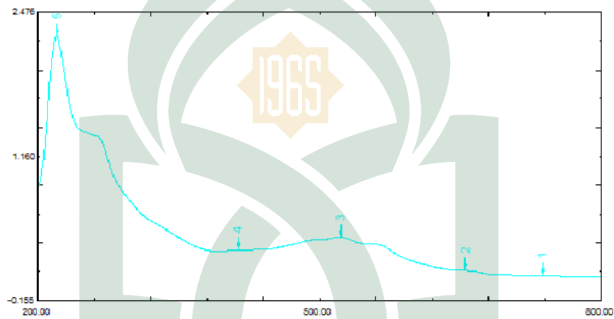
Gambar 2.9. Spektra karakteristik daun jati (Baharuddin, 2015 : 40)
