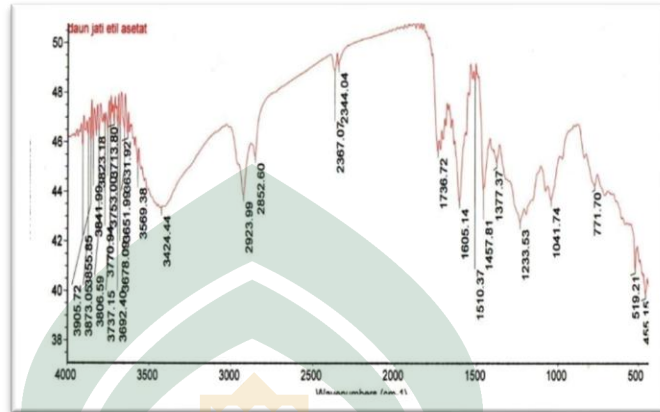
Gambar 4.5. Hasil serapan FTIR Ekstrak Etil Asetat Daun Jati
