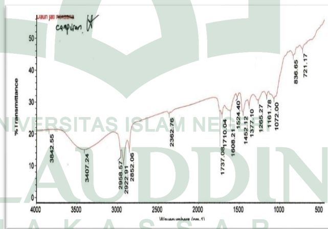
Gambar 4.7. Hasil serapan FTIR Ekstrak Gabungan Daun Jati
