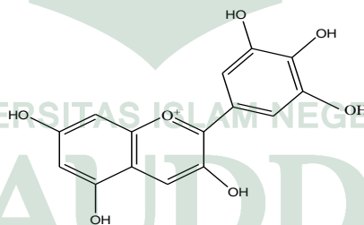
Gambar 2.3. Struktur Jenis Antosianin Sianidin ( Samber, 2013 : 1).
