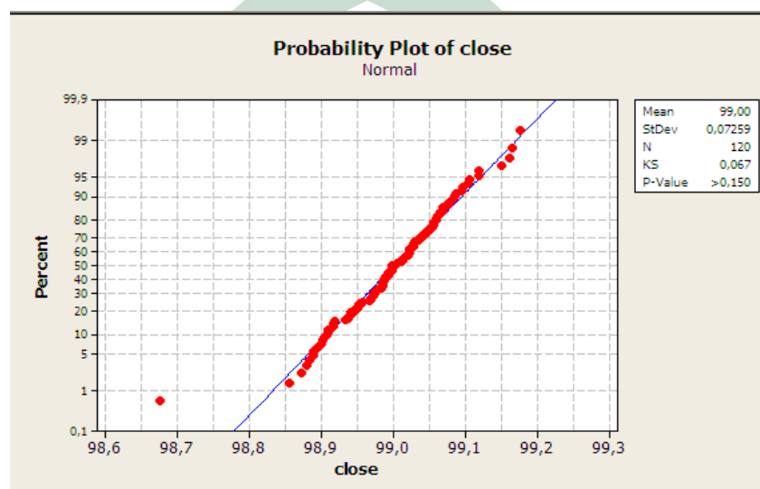
Gambar 4.2. Uji Normalitas Data Harga Penutupan PT Telekomunikasi Tbk
