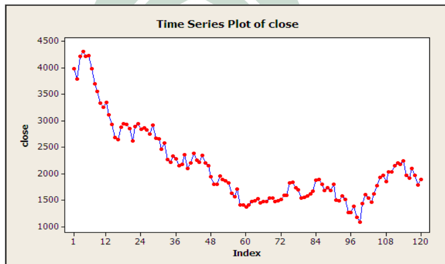
Gambar 4.1. Plot Data Harga Penutupan PT Telekomunikasi Tbk
