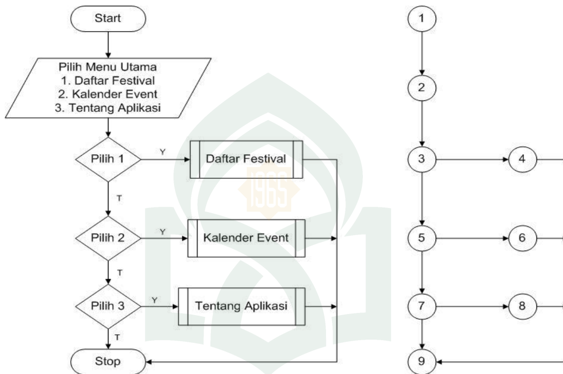
Gambar V. 22. Flowchart dan Flowgraph Menu Utama
