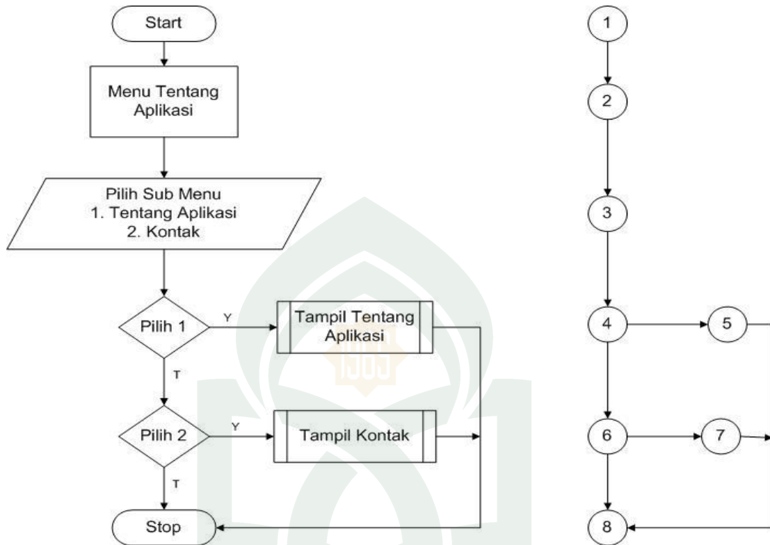
Gambar V. 25. Flowchart dan Flowgraph Tentang Aplikasi
