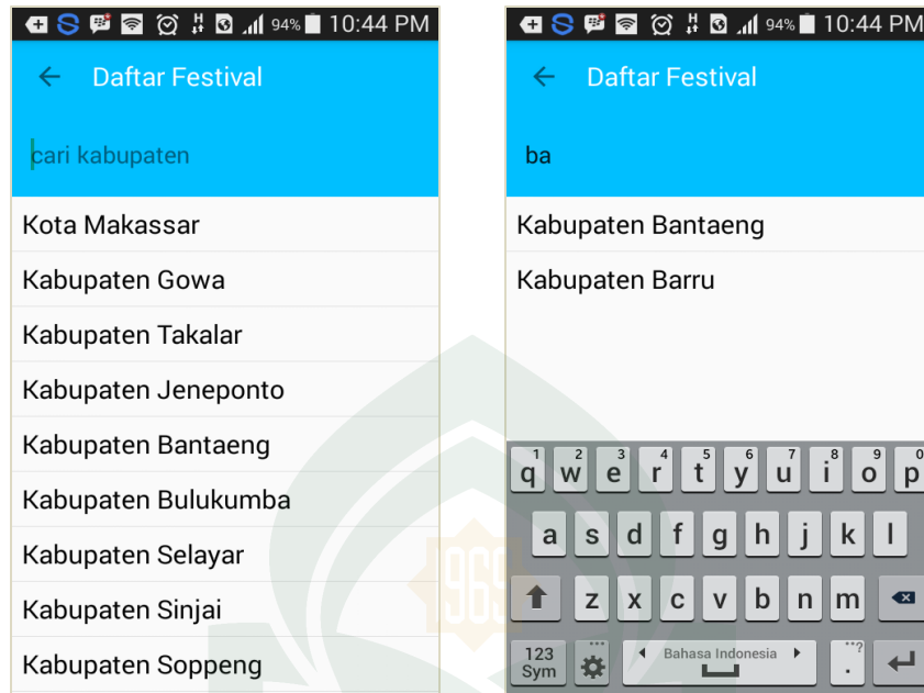
Gambar V. 3. Antarmuka Sub Menu Daftar Festival
