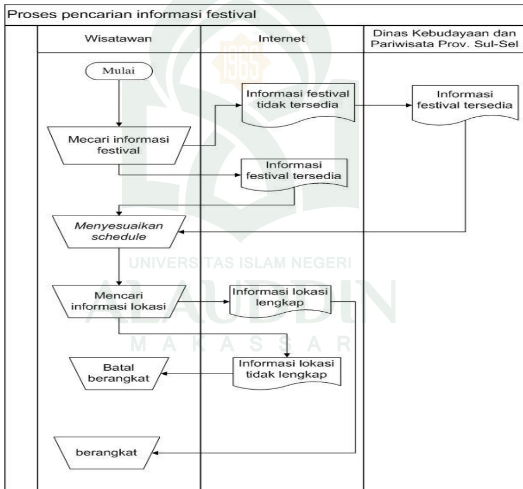
Gambar IV. 1. Flowmap sistem yang sedang berjalan
