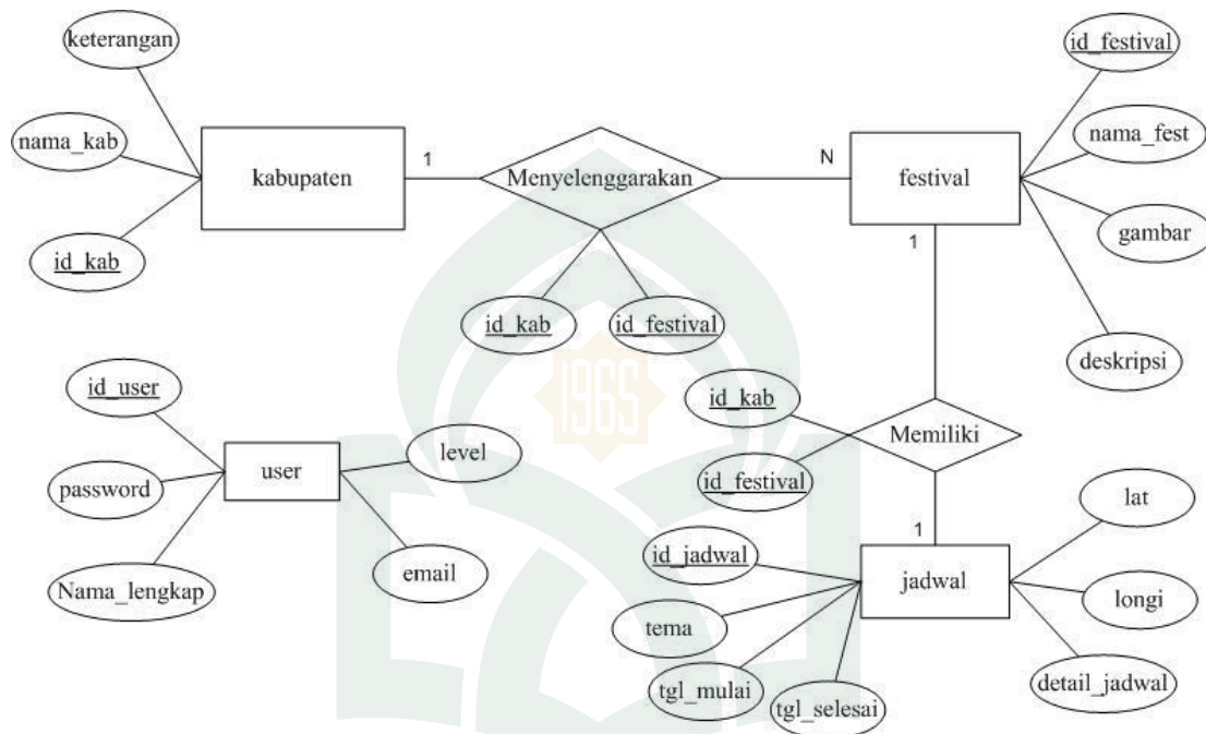
Gambar IV. 5. ERD Aplikasi Festival Budaya
