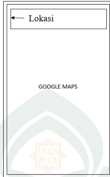
Gambar IV. 24. Tampilan Maps
