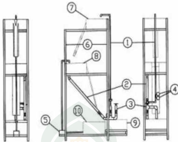
Gambar 2.16. Instalasi pompa hydram untuk percobaan
