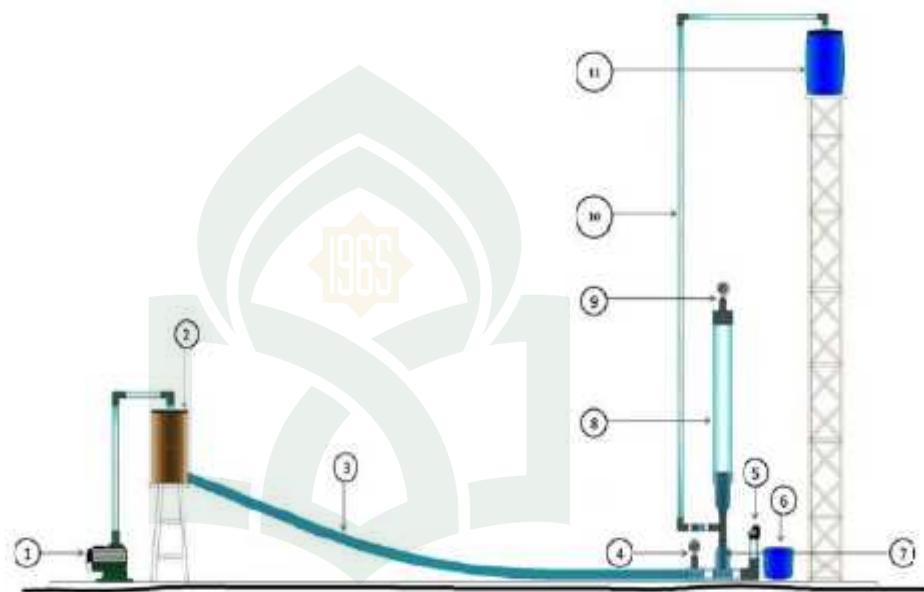
Gambar 2.8 Rangkaian pompa hidram
