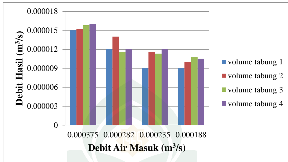
4.2. Grafik pengaruh debit air masuk terhadap debit hasil
