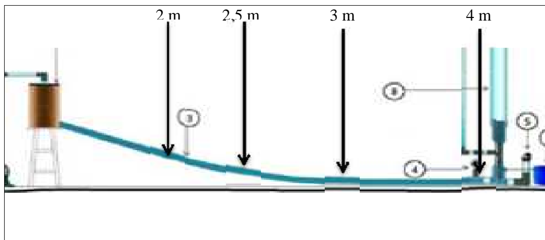
Gambar 4.2. Panjang pipa masuk pompa hydram
