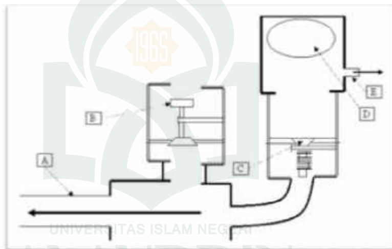
Gambar 2.12 Skema pompa hydram pada tahap penghantar
