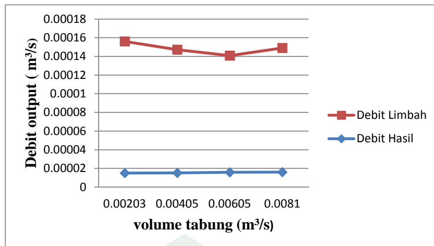
Grafik 4.1. Hubungan antara volume tabung dengan nilai debit hasil dan debit limbah
