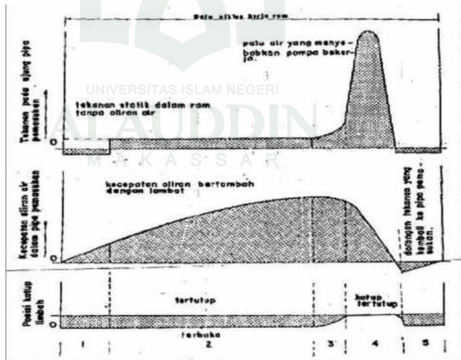
Gambar 2.14 Diagram satu siklus kerja pompa hydram
