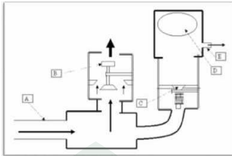
Gambar 2.10 Skema pompa hydram pada tahap akselerasi
