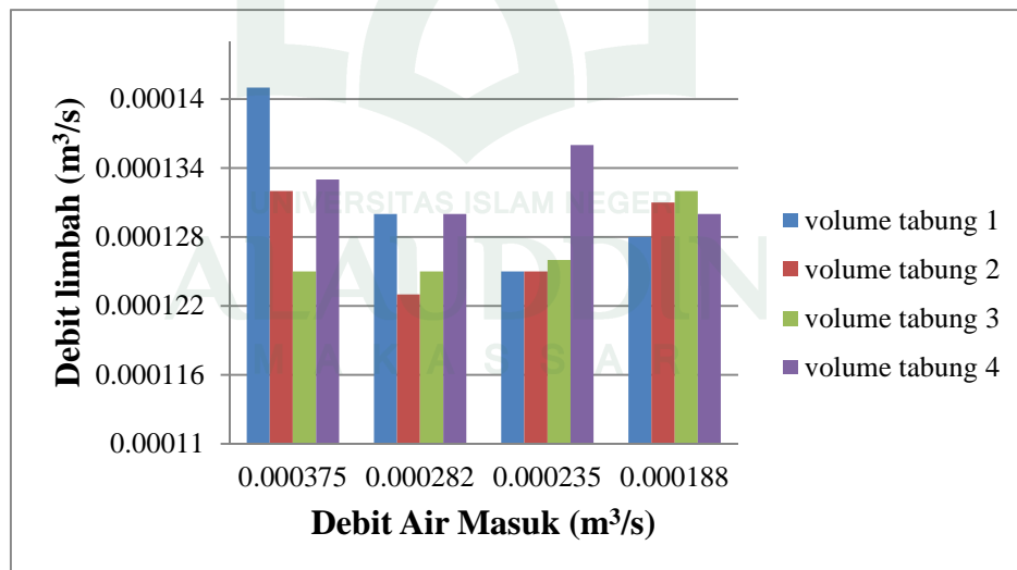
4.3. Grafik pengaruh debit air masuk terhadap debit limbah
