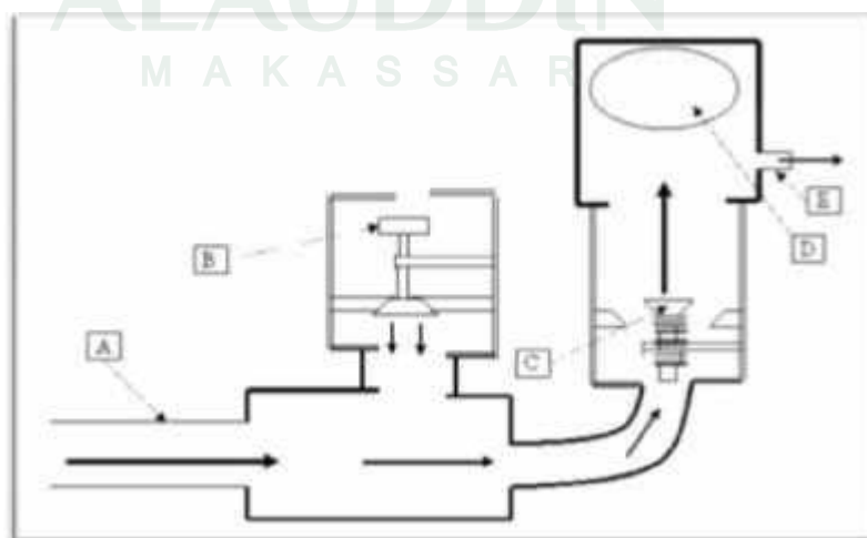
Gambar 2.11 Skema pompa hydram pada tahap kompresi
