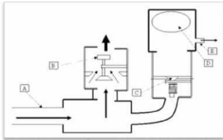
Gambar 2.13 Skema pompa hydram pada tahap rekoil
