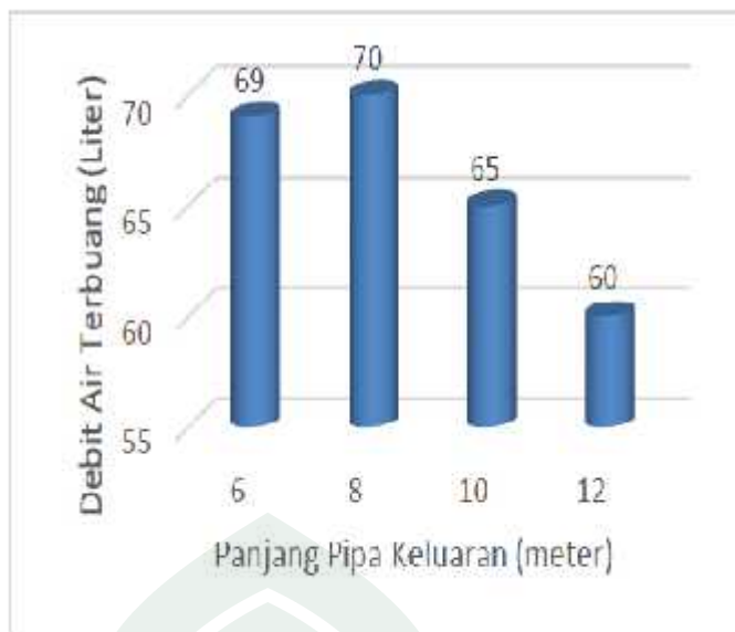
Gambar 2.17. Hubungan panjang pipa keluaran terhadap debit air terbuang
