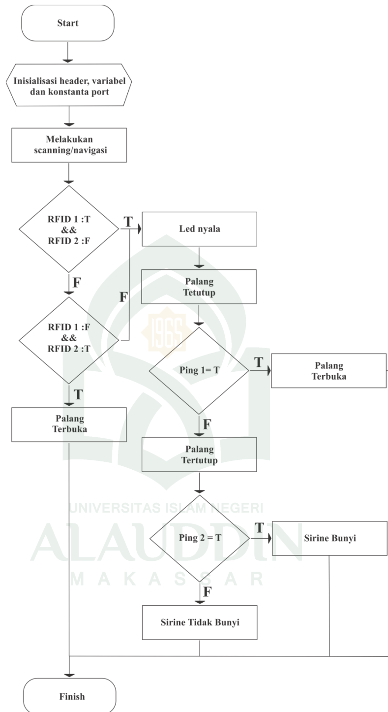
Gambar IV. 6 Flowchart Sistem Sirkulasi Bus pada Halte BRT
