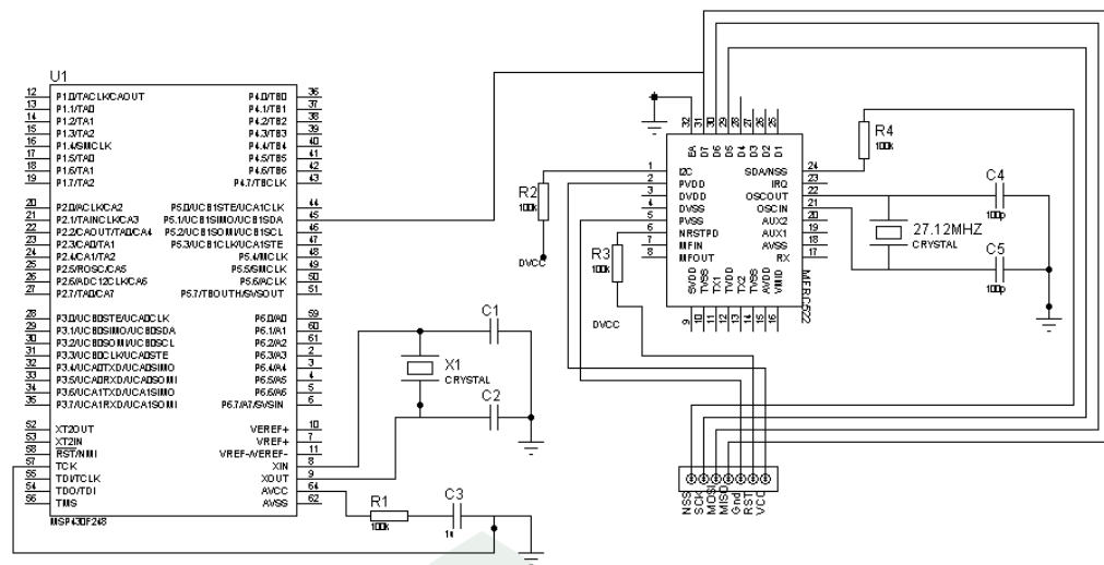
Gambar IV.3 Skema Modul RFID
