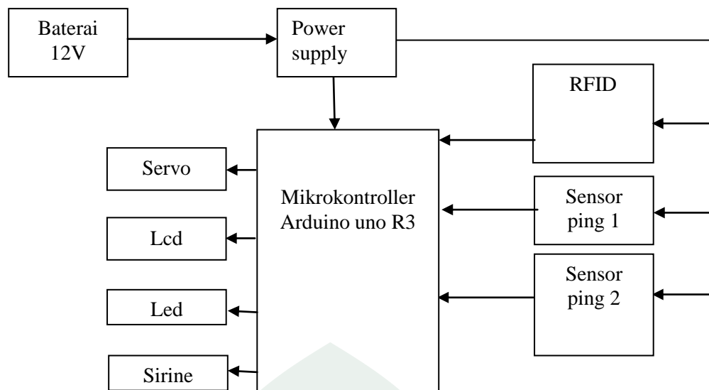
Gambar IV.1 Diagram Blok Sistem Kontrol Alat
