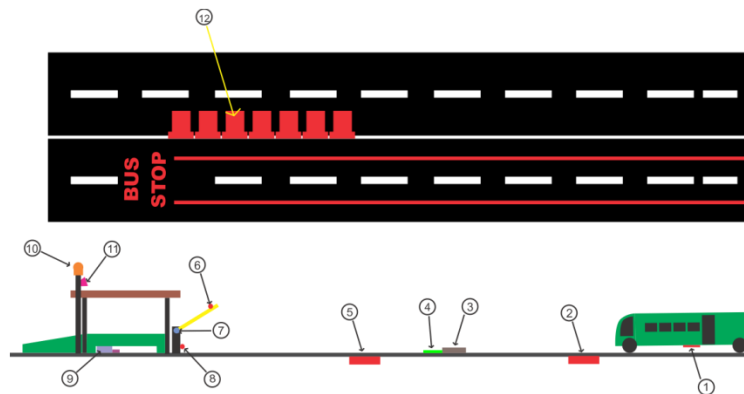
Gambar IV.2 Rancangan Sistem Sirkulasi Bus BRT
