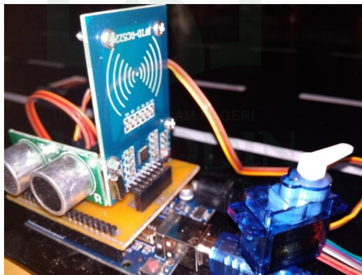
Gambar V. 4 Pengujian Menggunakan Servo
