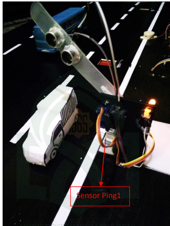
Gambar V. 7 kondisi Ketika Palang Mulai Tertutup
