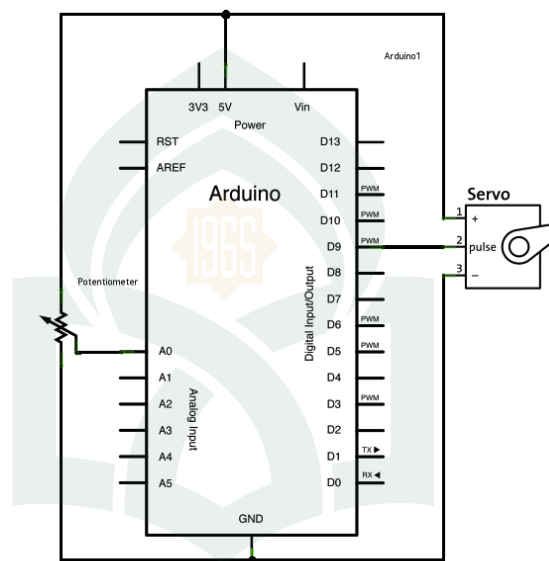
Gambar IV. 4 Rangkaian Motor Servo
