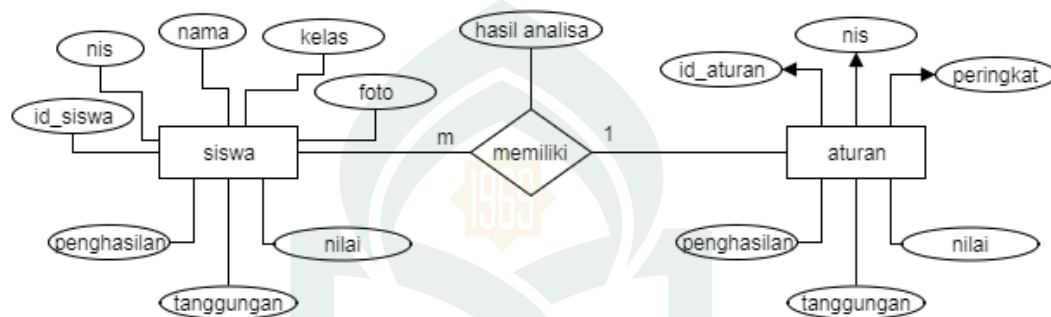
Gambar IV.18 Diagram ER
