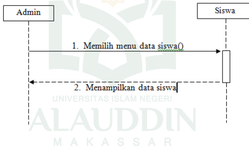
Gambar IV.6 Sequence diagram untuk data siswa
