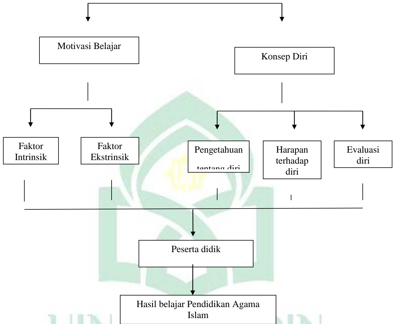
Gambar 2.1 Kerangka Pikir
