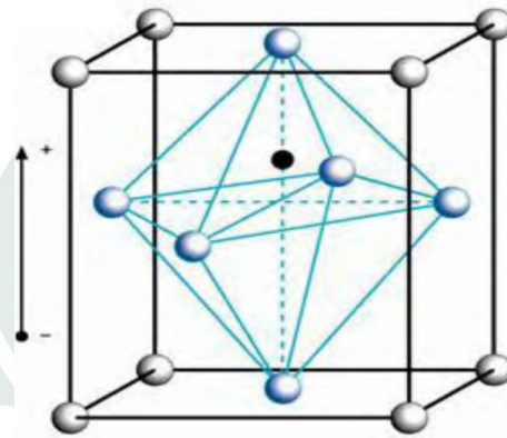
Gambar 2.4: Struktur perovskit \text{CaTiO}_3 (Sumber: Wahyuni, 2009: 2)
