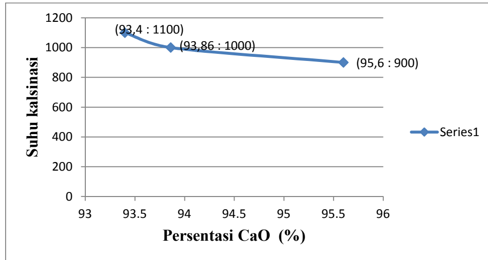
Gambar 4. 4 grafik hubungan antara suhu dengan kadar CaO
