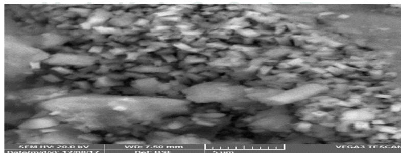
Gambar 4.1 hasil SEM dengan perbesaran 5 \mu\text{m} pada suhu 900 °C
