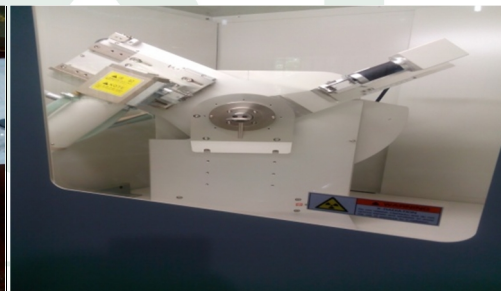
Analisis XRD
