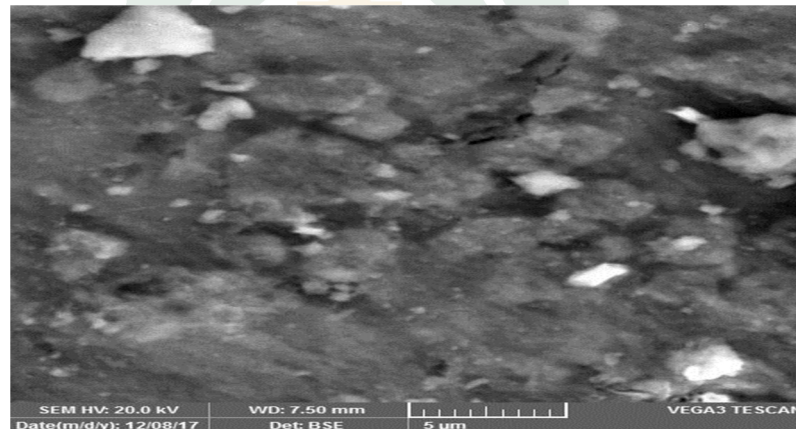
Gambar 4.3 hasil SEM dengan perbesaran 5 \mu\text{m} pada suhu 1100 ^{\circ}\text{C}
