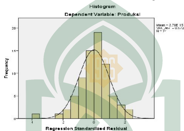
Gambar 2 Grafik Histogram
