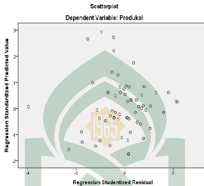
Gambar 4 Uji Heteroskedastisitas
