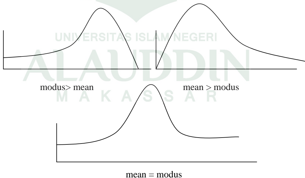
Gambar 2.1 Skewness (Kecondongan)
