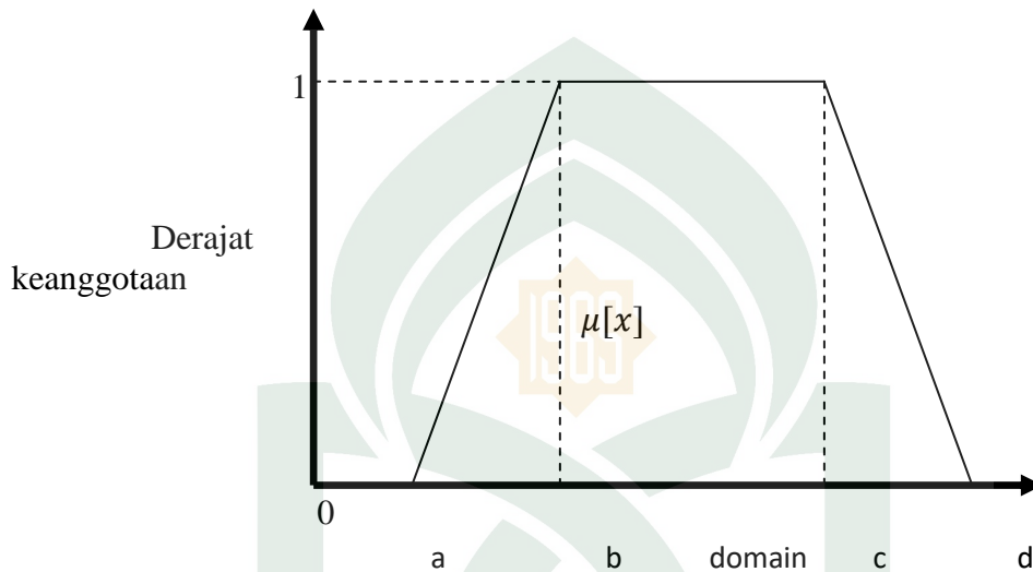
Gambar 2.6 Kurva trapesium
