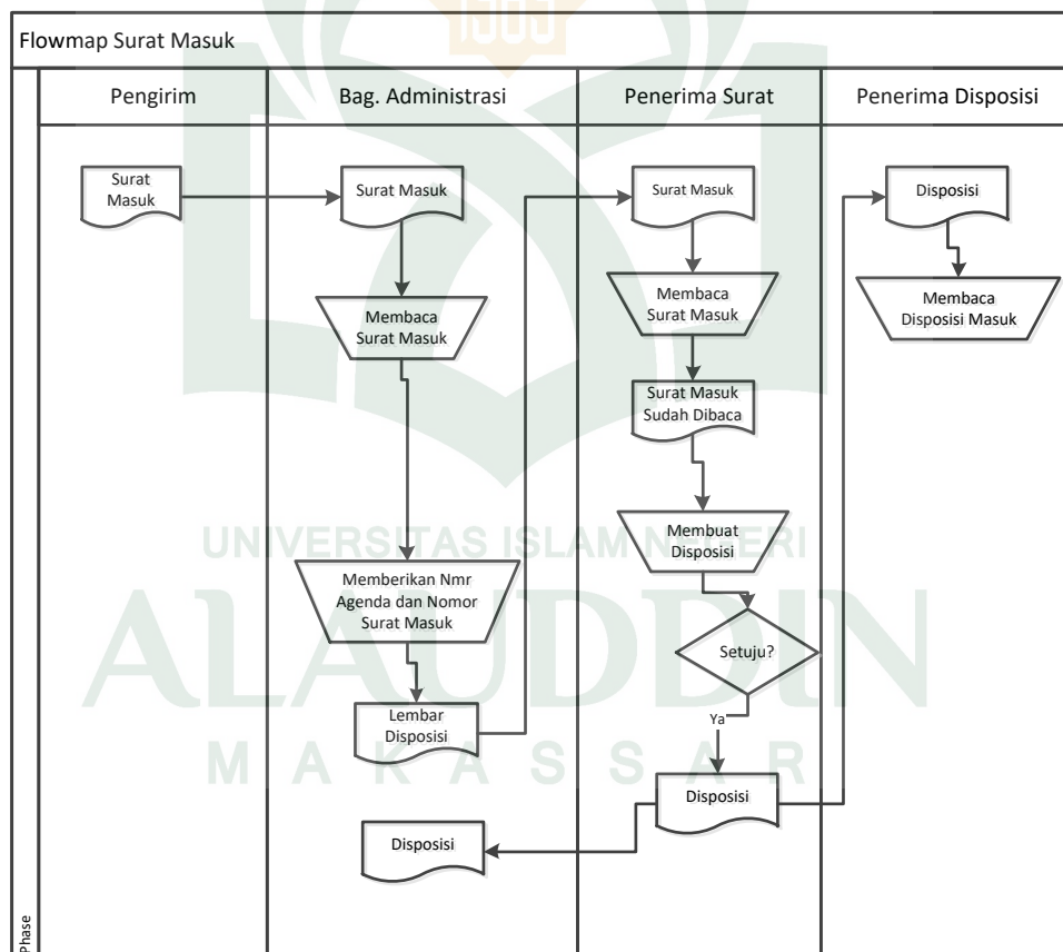
Gambar IV. 1 Sistem proses surat masuk yang sedang berjalan
