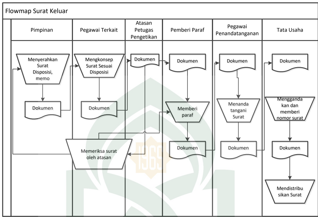
Gambar IV. 3 Sistem proses surat keluar yang sedang berjalan
