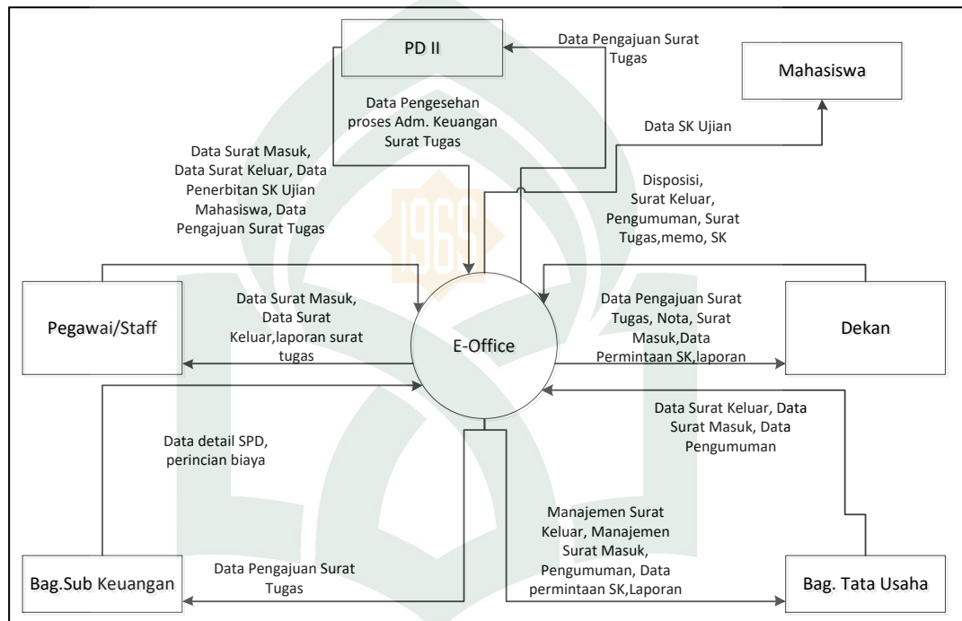
Gambar IV. 5 Konteks Diagram Sistem
