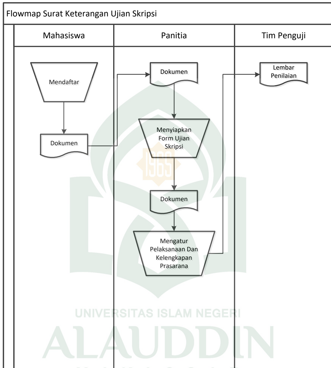
Gambar IV. 4 Sistem proses ujian skripsi yang sedang berjalan
