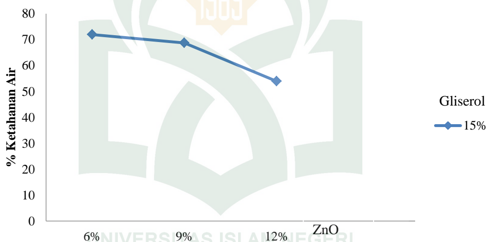
Gambar 4.2. Grafik Hasil Uji Ketahanan Plastik Biodegradable Terhadap Air dari Pati Biji Nangka dengan Variasi Konsentrasi ZnO dan Gliserol 15%
