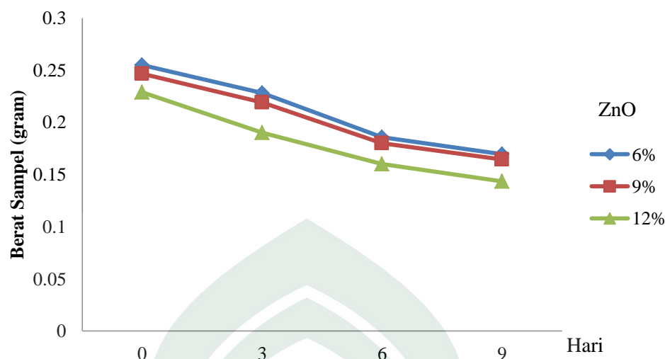
Gambar 4.3. Grafik Hasil Uji Biodegradabilitas Plastik Biodegradable
