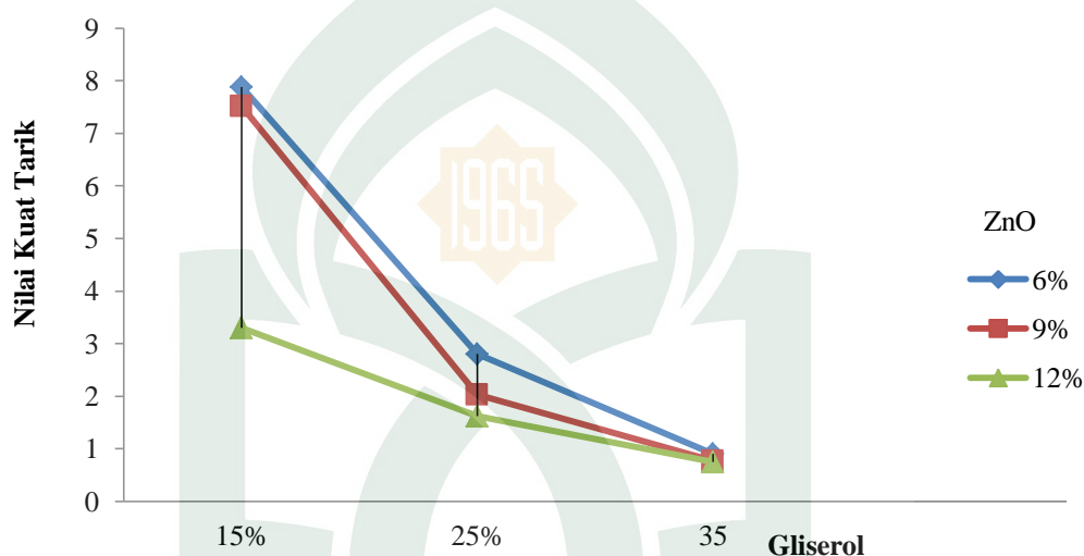
Gambar 4.1. Grafik Hasil Uji Kuat Tarik dari Pati Biji Nangka dengan Variasi Konsentrasi Gliserol dan ZnO
